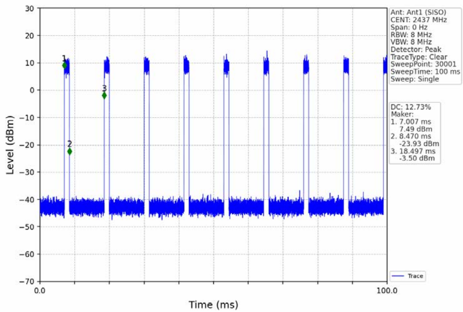
802.11ax(HEW20)_MCH_2437MHz_RU242_Left_Ant1 (SISO)_NTNV
