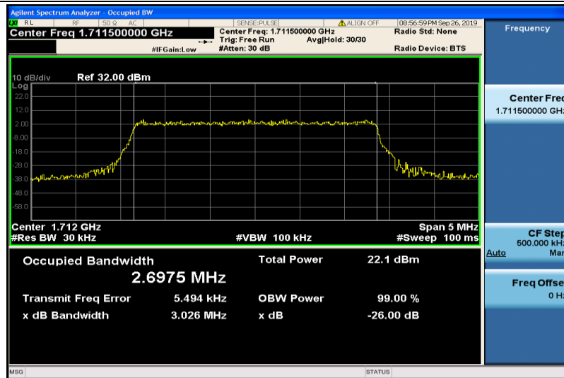
Band4-3MHz-QPSK-19965-15RB#0-2.6975
