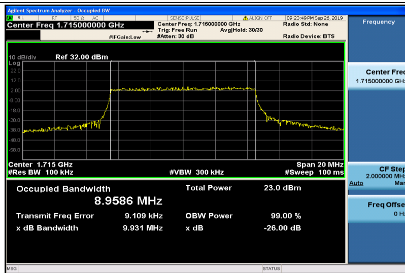
Band4-10MHz-QPSK-20000-50RB#0-8.9586
