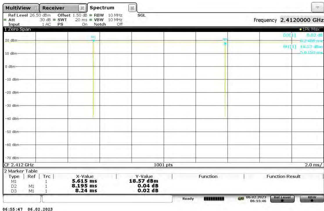
11G_Ant0_2412
