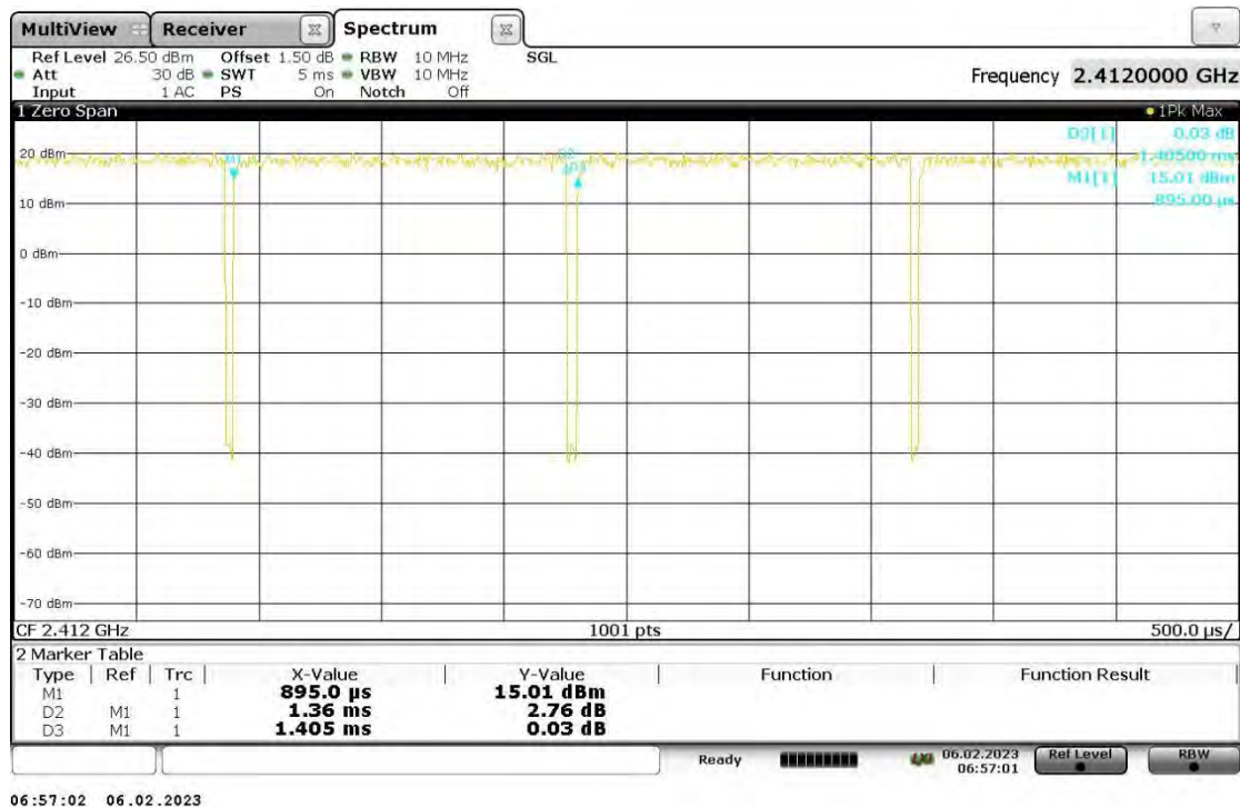
11N20_Ant0_2412
