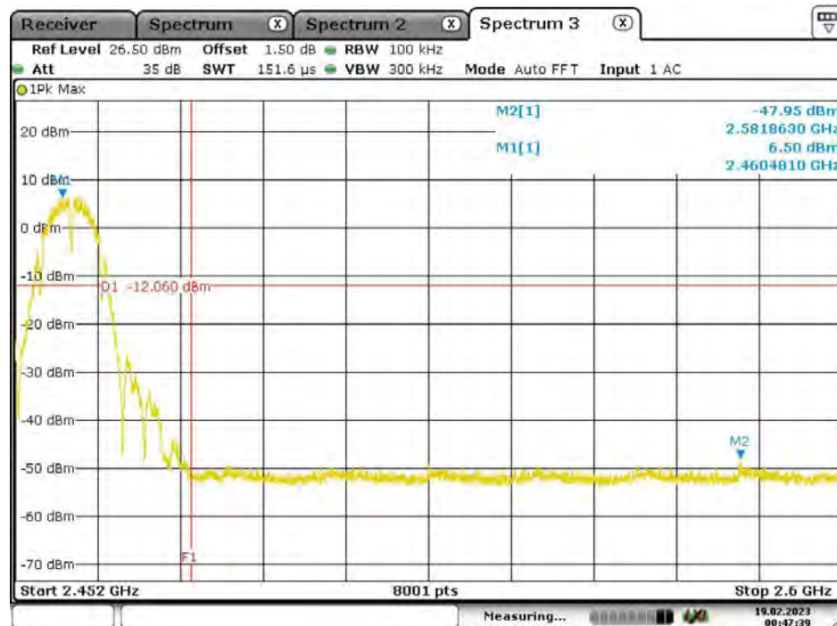
11B_Ant0_High_2462
