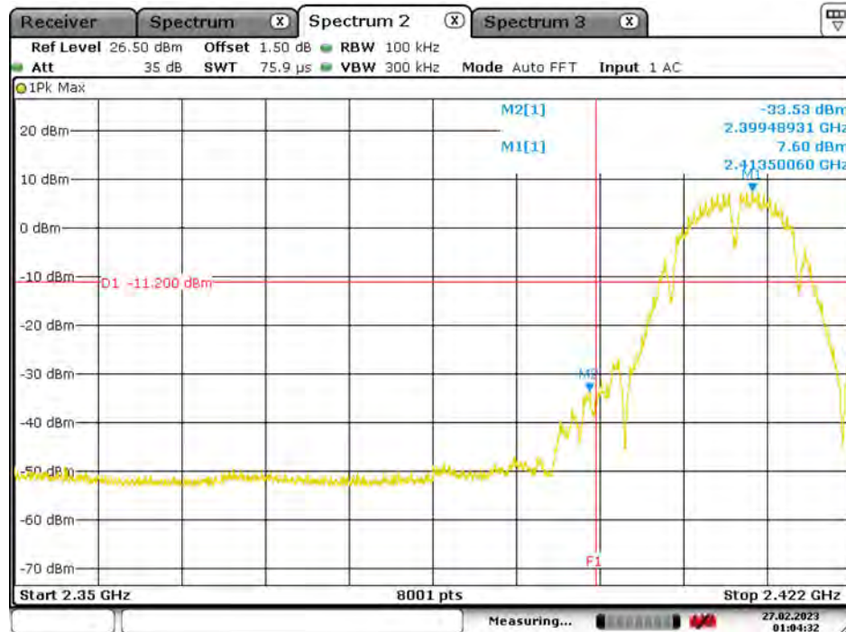
11B_Ant0_Low_2412
