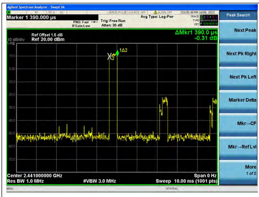
(DH1, 8-DPSK)
