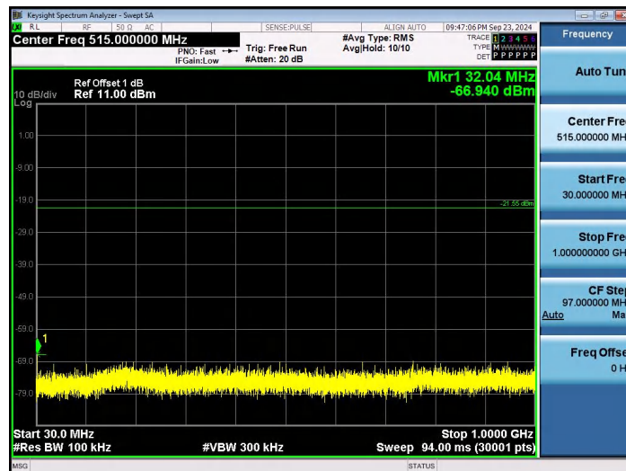
BLE_2M-Ant1-2402-30~1000-PASS
