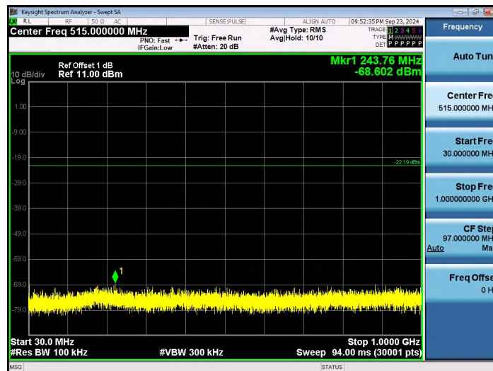
BLE_2M-Ant1-2440-30~1000-PASS
