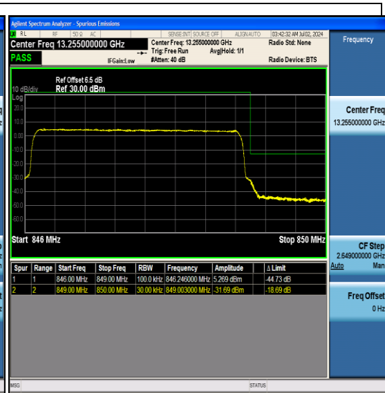
Band5_3MHz_64QAM_20635_15RB#0
