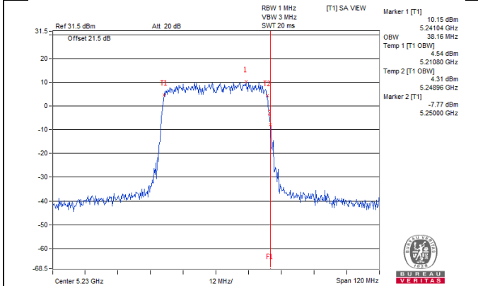
802.11ax (HE40) Chain 2 / CH46
