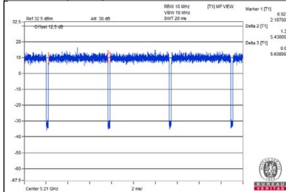
802.11ax (HE80)
