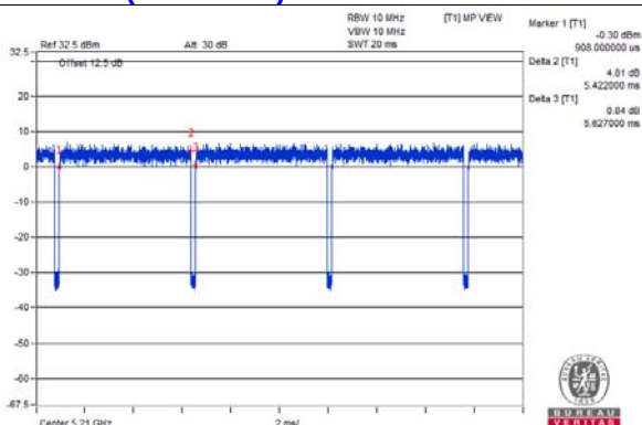
802.11ac (VHT80+80)
