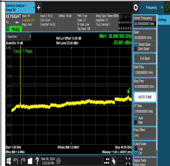
NTNV-N77-3700-3980-PC2-30-60-H-DFT-QPSK- Edge 1RB Left-Ant1-PASS
