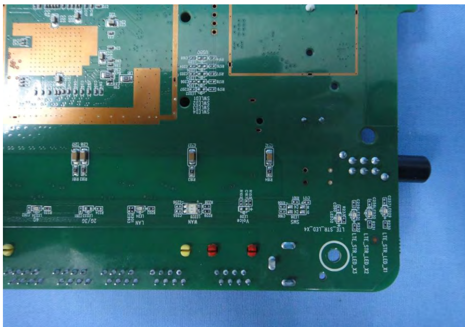
EUT Photo (4)
