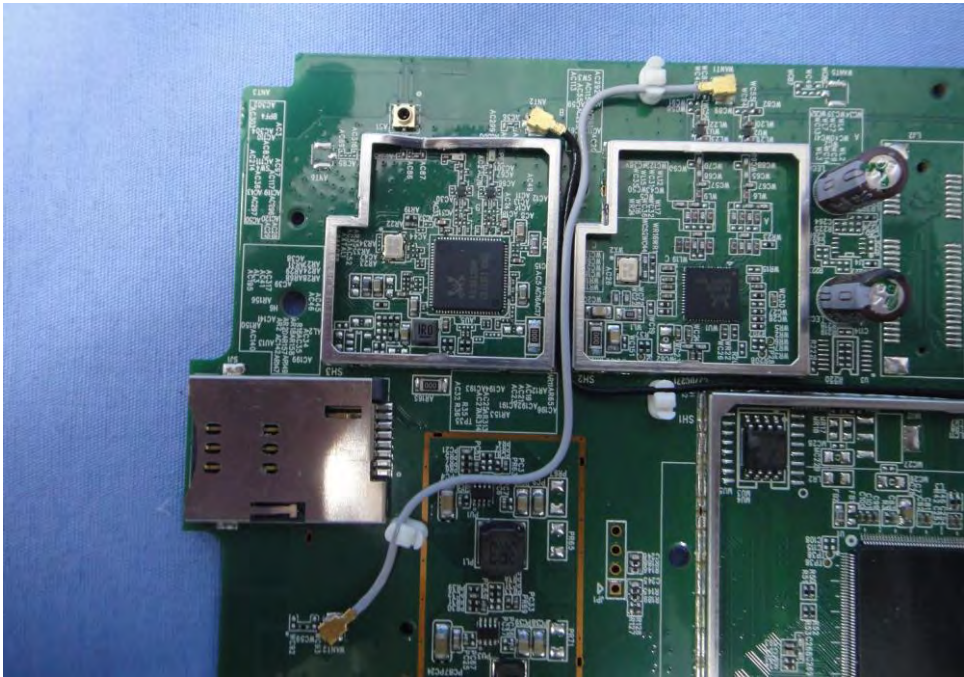
EUT Photo (15)
