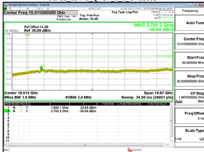
Band2 15kHz QPSK 1 0 CH18900
