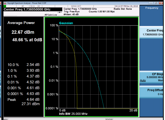
16QAM-132072
