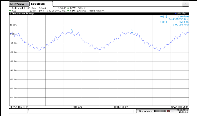
GFSK
