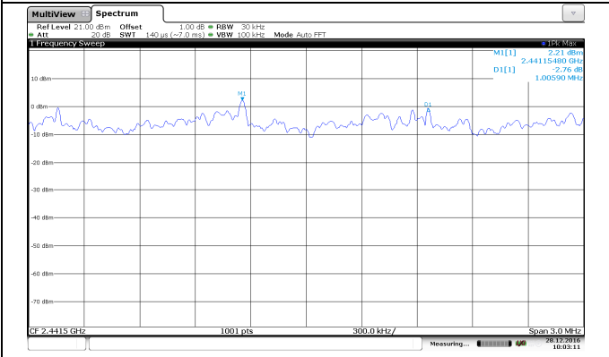
8DPSK
