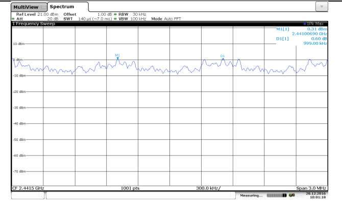
\pi/4 DQPSK
