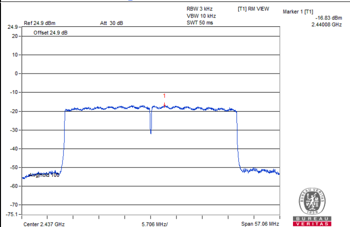
802.11be (EHT40) Beamforming / Chain 1 : CH 6
