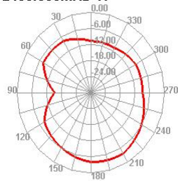
2400.000MHz H
