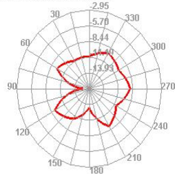
2400.000MHz E2
