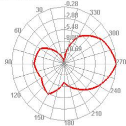
2500.000MHz E1
