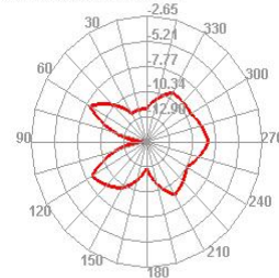
2410.000MHz E2
