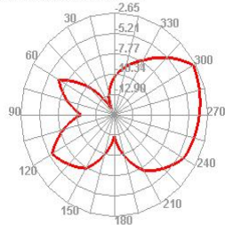
2410.000MHz E1
