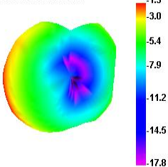
2450.000MHz
