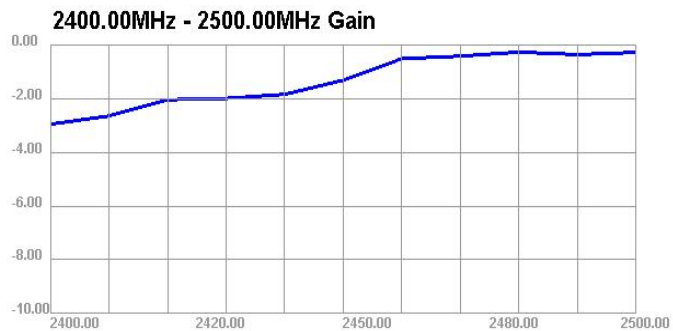
2400.000MHz H
