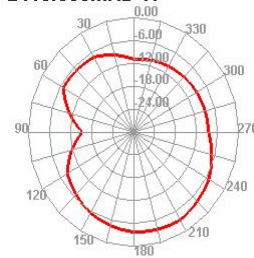
2410.000MHz H
