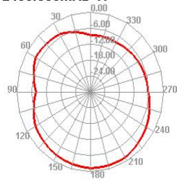
2450.000MHz H
