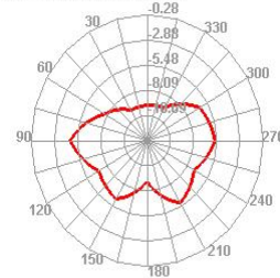
2500.000MHz E2
