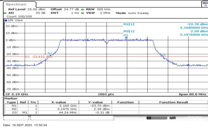
11AC40MIMO_Ant4_5190
