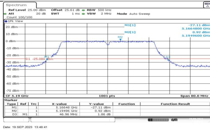
11AC40MIMO_Ant1_5190
