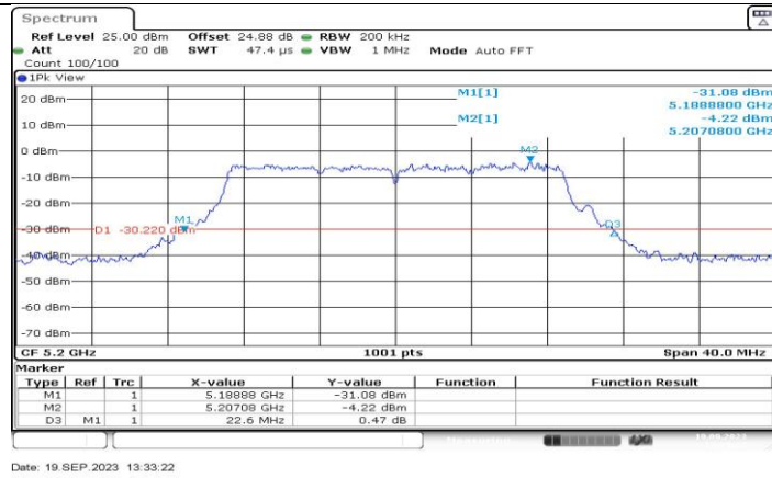
11AC20MIMO_Ant3_5200
