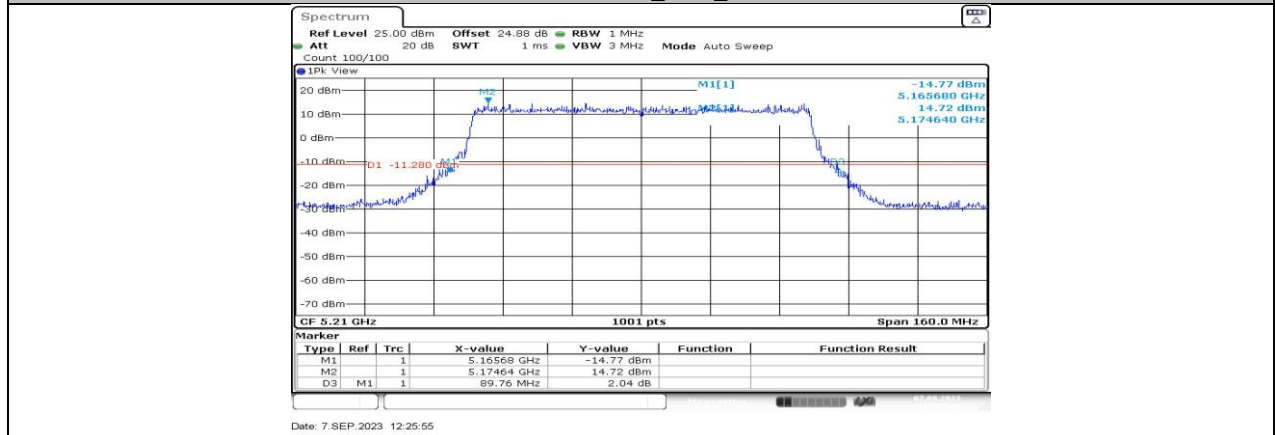
11BE80MIMO_Ant3_5210
