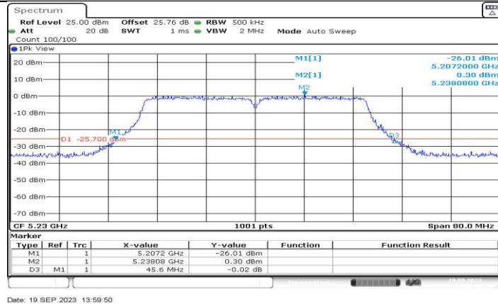
11AC40MIMO_Ant2_5230
