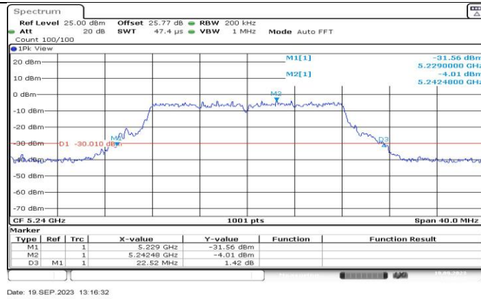
11A-CDD_Ant2_5240
