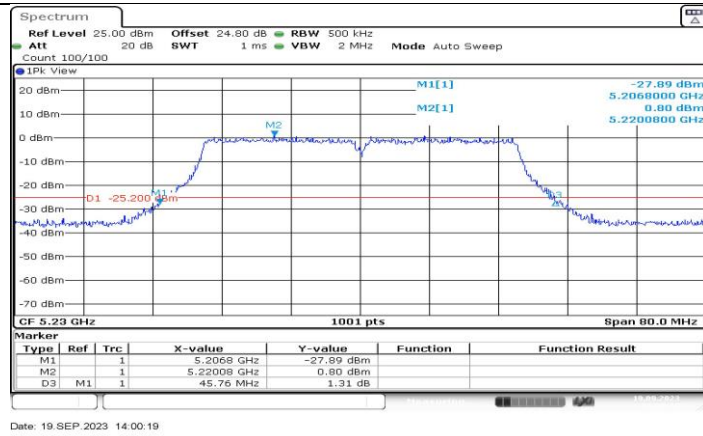
11AC40MIMO_Ant3_5230
