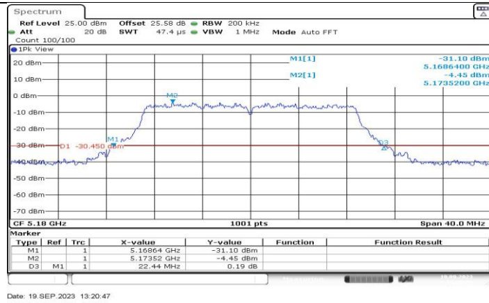
11AC20MIMO_Ant1_5180
