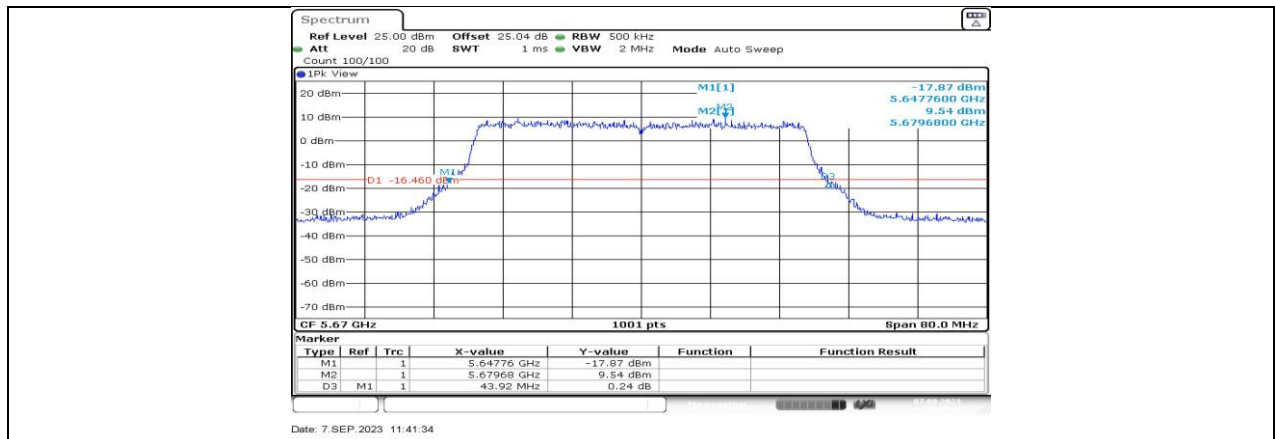
11BE40MIMO_Ant4_5670
