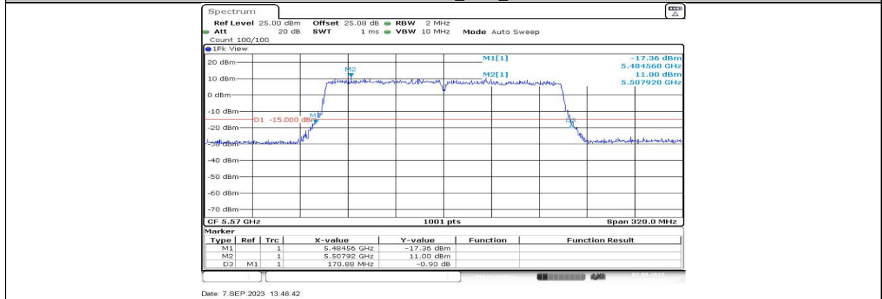
11BE160MIMO_Ant4_5570
