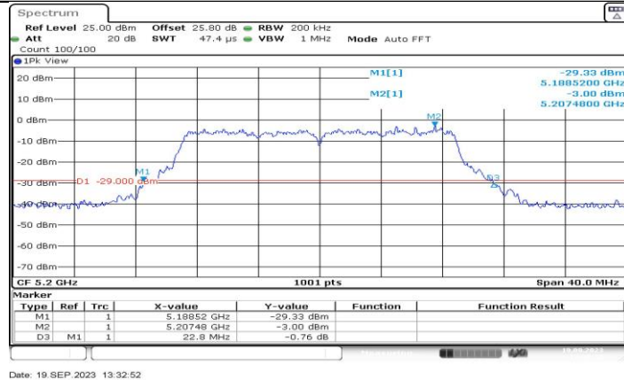
11AC20MIMO_Ant2_5200
