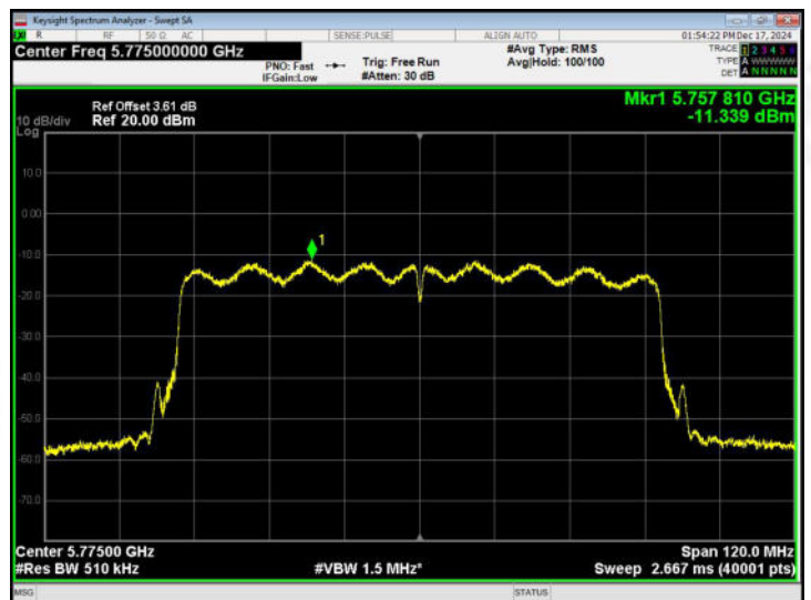
802.11ac80 - CH 155
