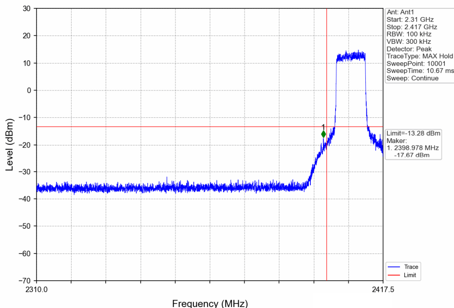
10MHz BW_LCH_2407.5MHz_Ant1_NTNV
