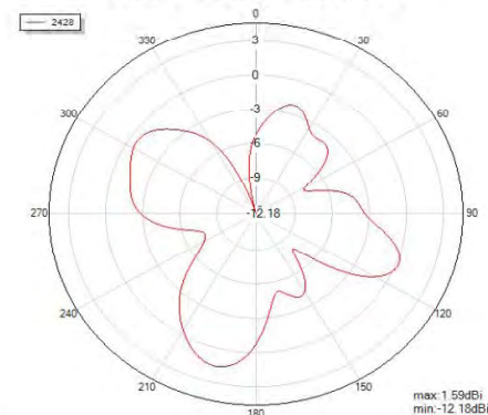
Theta=90 freq=2428MHz
