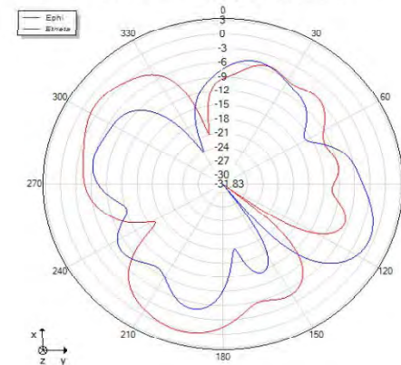
Theta=90 freq=2428MHz
