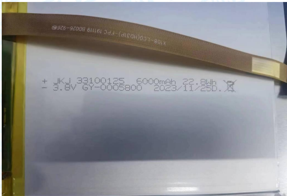
Photo 10 Battery parameters
