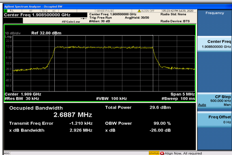
Band2-3MHz-QPSK-19185-15RB#0-2.6887
