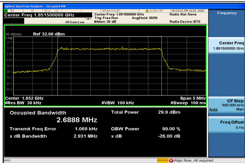
Band2-3MHz-QPSK-18615-15RB#0-2.6888
