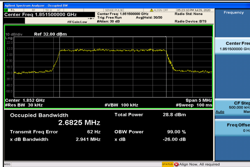
Band2-3MHz-16QAM-18615-15RB#0-2.6825
