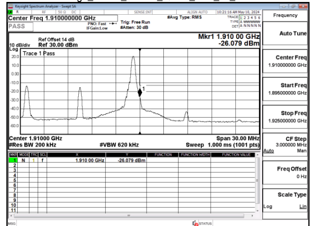
Band Edge_Band2_15MHz_QPSK_RB1_74_CH19125
