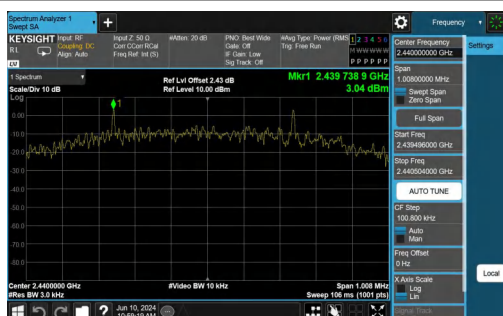
BLE_500K-Ant1-2440-PASS
