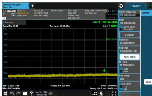
BLE_500K-Ant1-2440-30~1000-PASS
