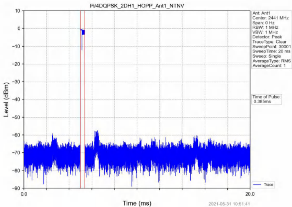
Pi/4DQPSK_2DH1_HOPP_Ant1_NTNV
