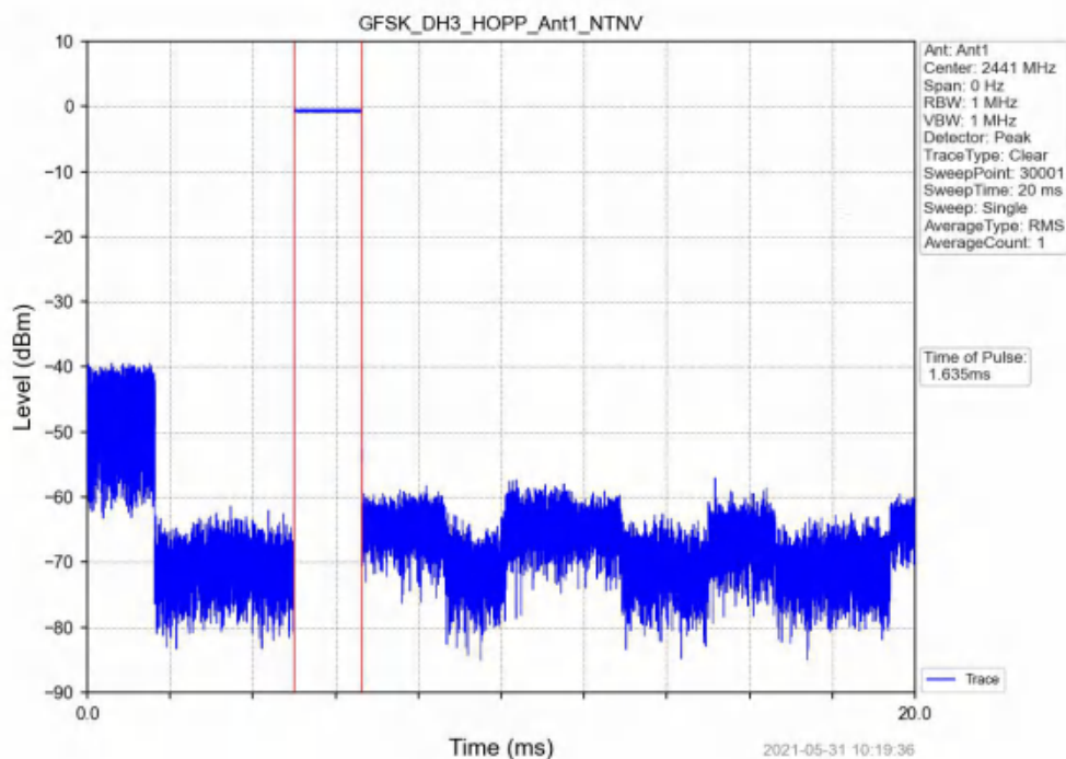
GFSK_DH3_HOPP_Ant1_NTNV
