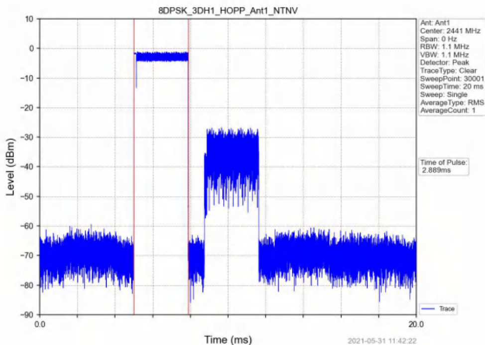
8DPSK_3DH1_HOPP_Ant1_NTNV
