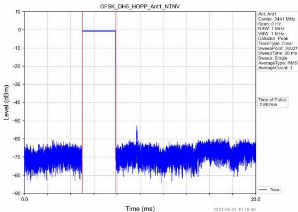
GFSK_DH5_HOPP_Ant1_NTNV
