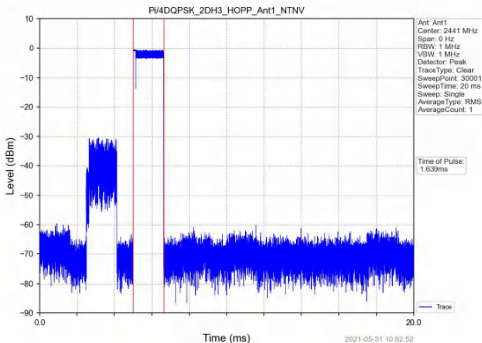
Pi/4DQPSK_2DH3_HOPP_Ant1_NTNV
