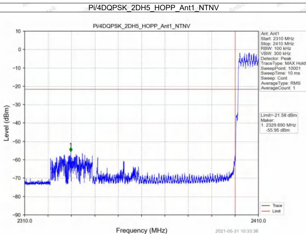
Pi/4DQPSK_2DH5_HOPP_Ant1_NTNV
