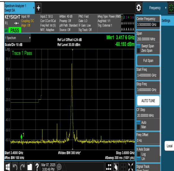
NTNV-N77-3450-3550-PC2-30-50-L-DFT-QPSK- Edge 1RB Right-Ant1-PASS
