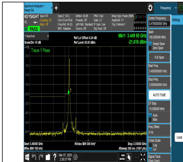
NTV-N77-3450-3550-PC2-30-10-L-DFT-QPSK- Edge 1RB Left-Ant1-PASS
