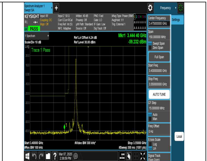
NTV-N77-3450-3550-PC2-30-10-L-DFT-QPSK- Edge 1RB Right-Ant1-PASS
