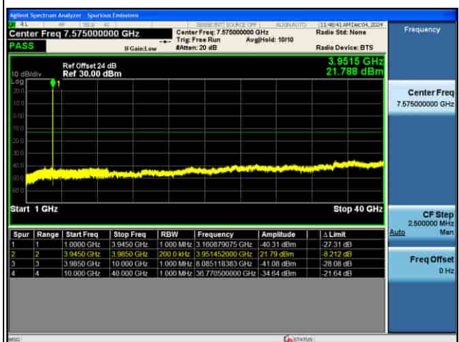
CSE_5G_n77(N)_30KHz_QPSK_30M CH664332_1RB@1_
