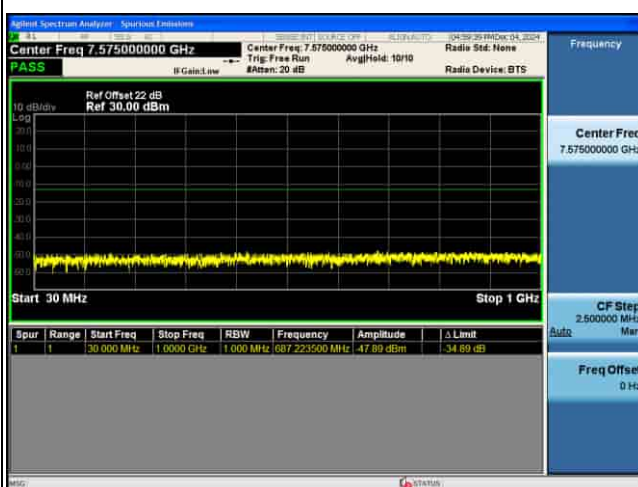
CSE_5G_n77(N)_30KHz_.PI2-BPSK_90M CH662332_1RB@1
