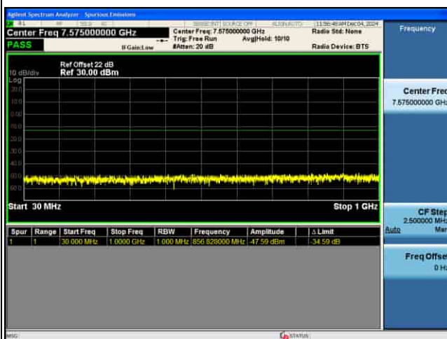
CSE_5G_n77(N)_30KHz_.PI2-BPSK_30M CH664332_1RB@1
