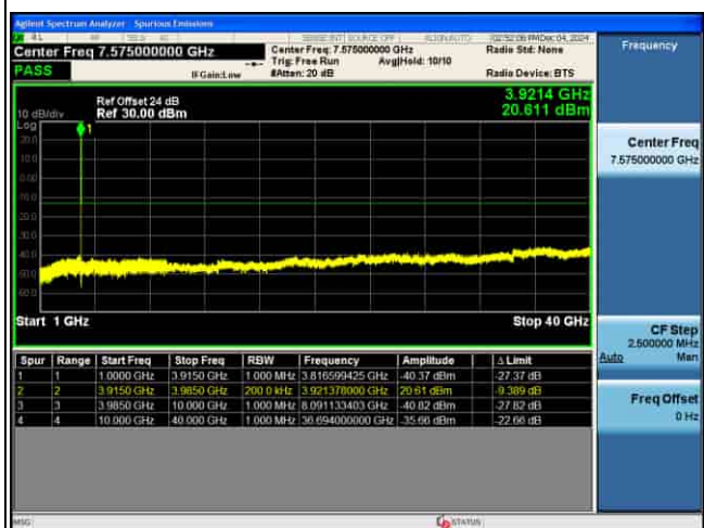
CSE_5G_n77(N)_30KHz_.PI2-BPSK_60M CH663332_1RB@1_
