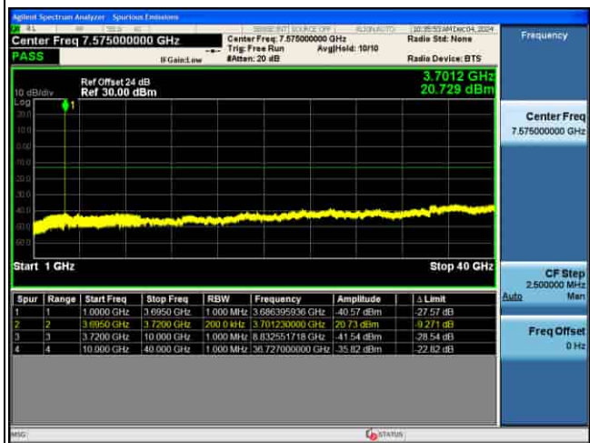
CSE_5G_n77(N)_30KHz_.PI2-BPSK_15M CH656000_1RB@1_
