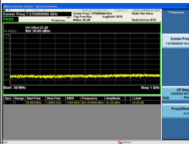
CSE_5G_n77(N)_30KHz_.PI2-BPSK_60M CH663332_1RB@1
