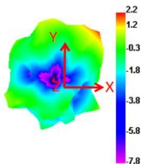
2450.000MHz
