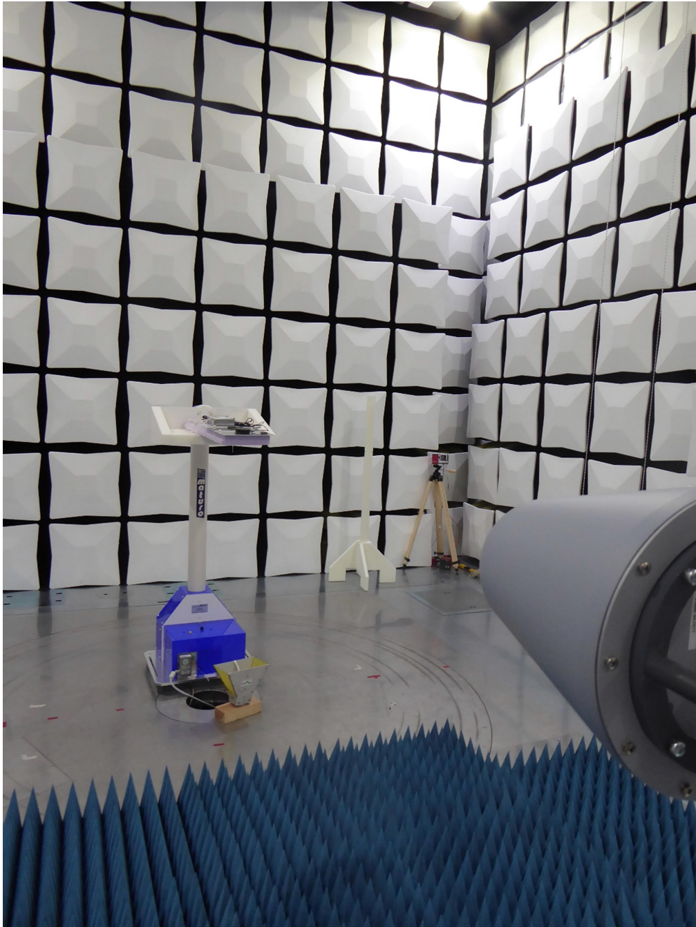
Test setup 1 - 18GHz
