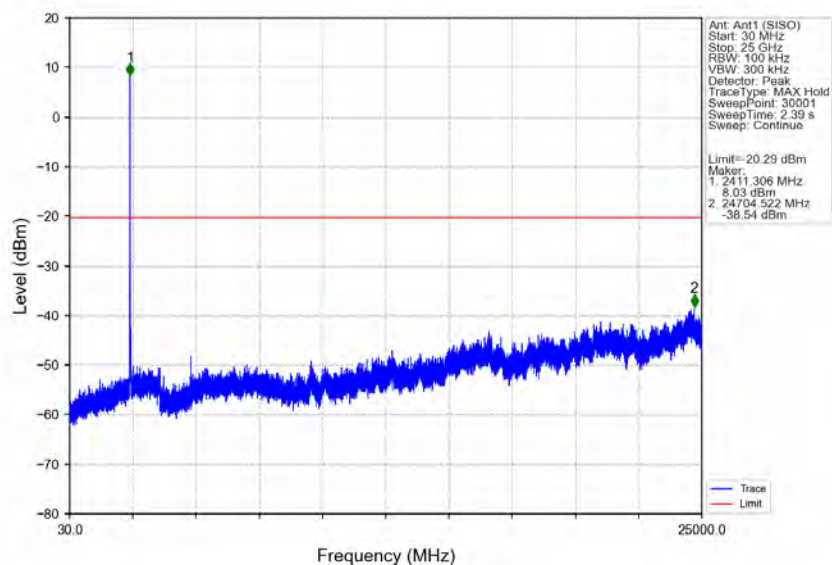
802.11b_LCH_2412MHz_Ant1 (SISO)_NTNV
