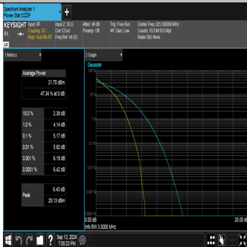
Band26(824-849)-3MHz-QPSK-26805-15RB#0-PASS
