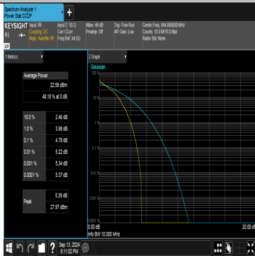
Band26(824-849)-10MHz-QPSK-26990-1RB#0-PASS
