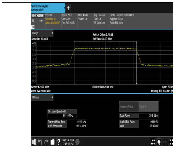
Band26(824-849)-10MHz-QPSK-26840-50RB#0-PASS
