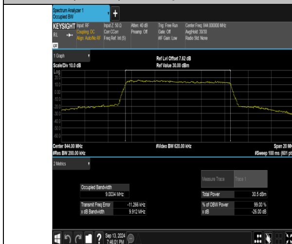
Band26(824-849)-10MHz-QPSK-26990-50RB#0-PASS
