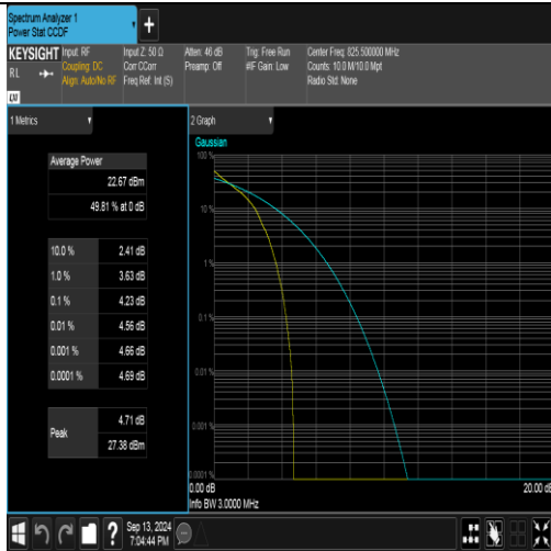
Band26(824-849)-3MHz-QPSK-26805-1RB#0-PASS
