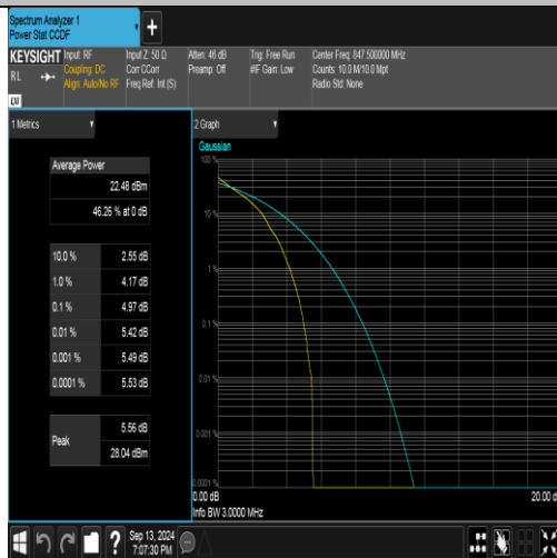
Band26(824-849)-3MHz-QPSK-27025-1RB#0-PASS
