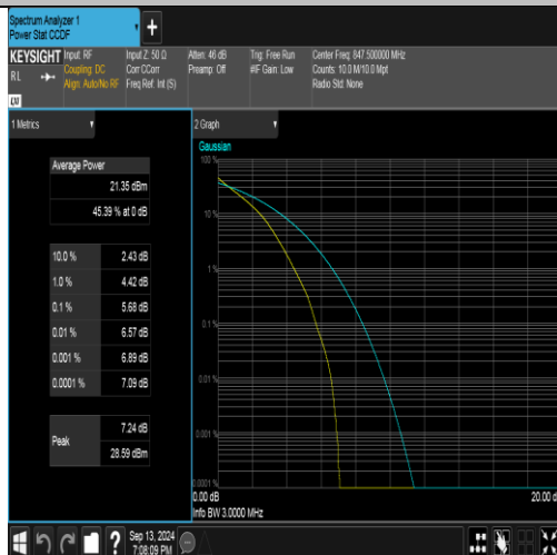
Band26(824-849)-3MHz-QPSK-27025-15RB#0-PASS
