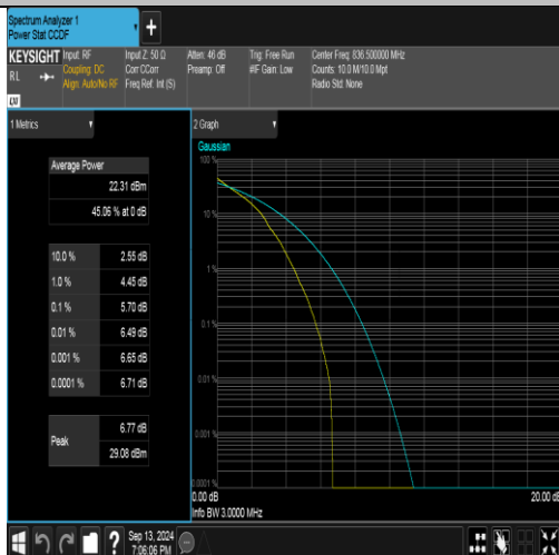
Band26(824-849)-3MHz-QPSK-26915-1RB#0-PASS
