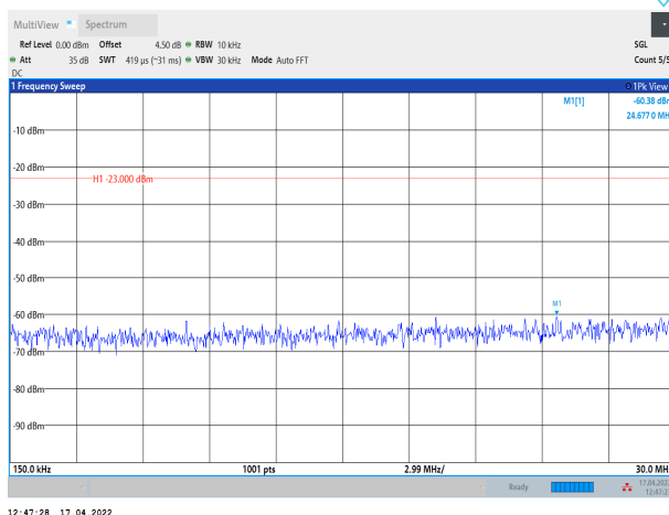
Band26-10MHz-QPSK-26740-1RB#0-Range2:0.15~30MHz
