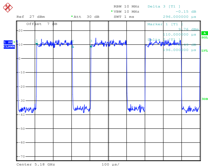
802.11a Antenna 1
