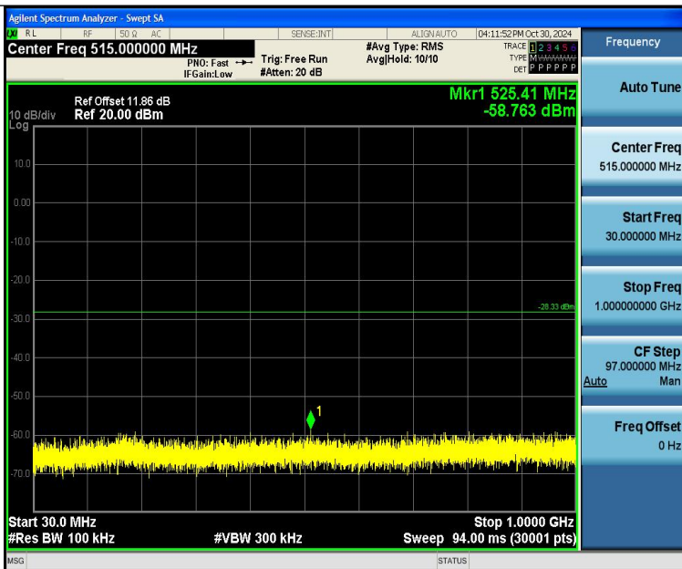
11G-Ant1-2462-30~1000-PASS
