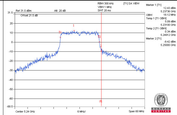
802.11ac(VHT20)_Chain2 / CH48
