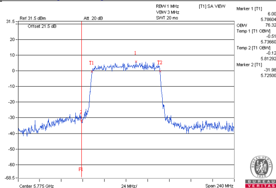
802.11ac(VHT80)_Chain2 / CH155
