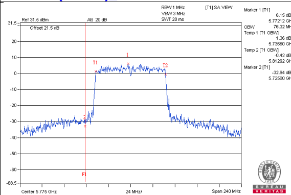
802.11ac(VHT80)_Chain1 / CH155
