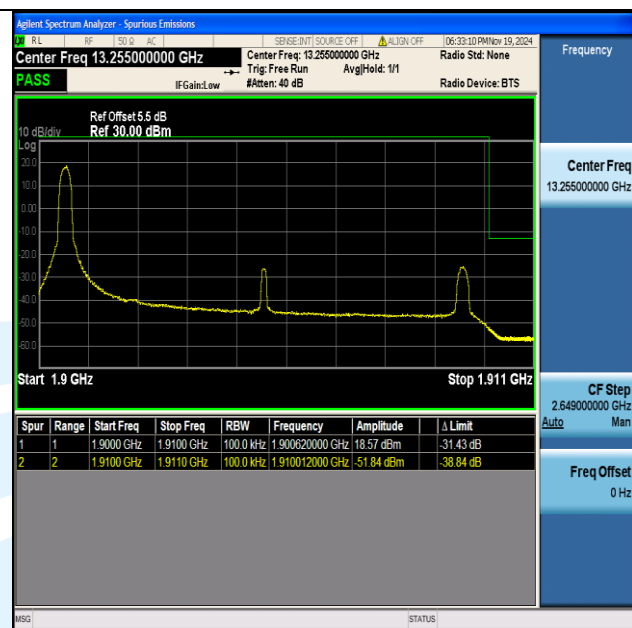
Band2 10MHz 16QAM 19150 1RB#0
