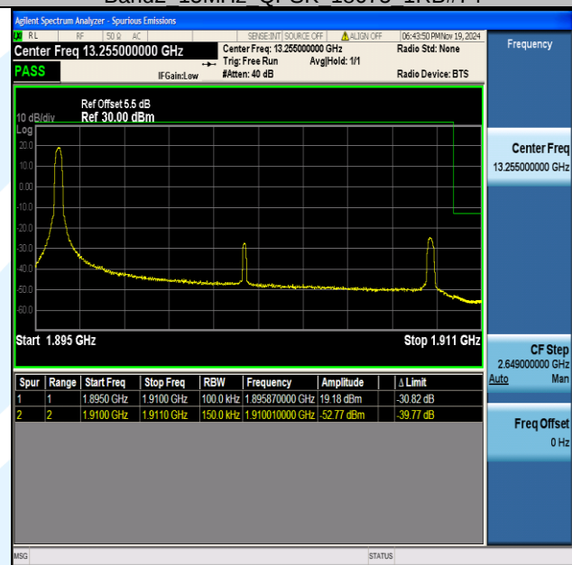
Band2 15MHz QPSK 19125 1RB#0
