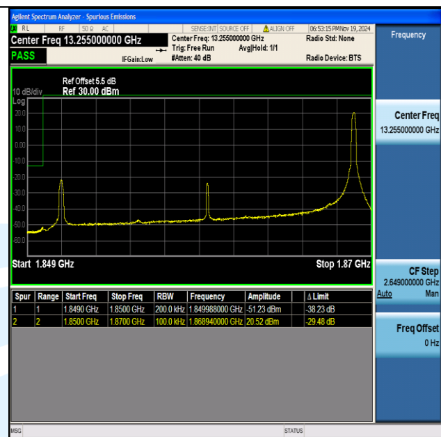
Band2 20MHz QPSK 18700 1RB#99
