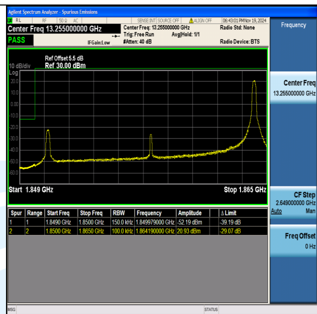
Band2 15MHz QPSK 18675 1RB#74
