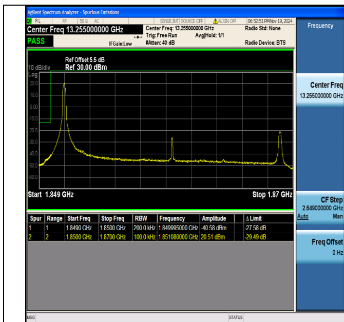
Band2 20MHz QPSK 18700 1RB#0
