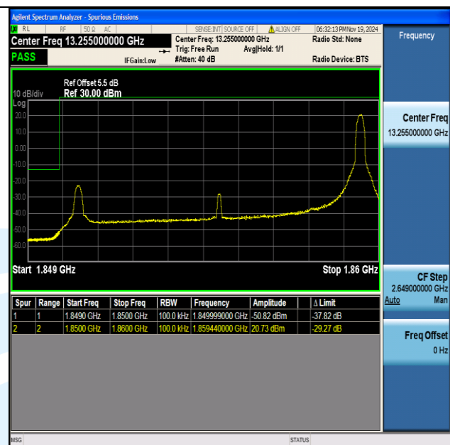
Band2 10MHz QPSK 18650 1RB#49
