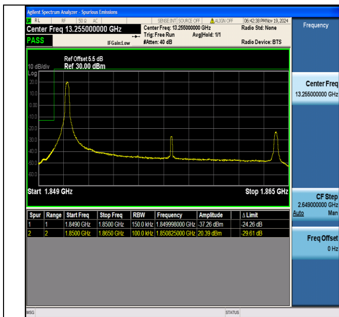
Band2 15MHz QPSK 18675 1RB#0
