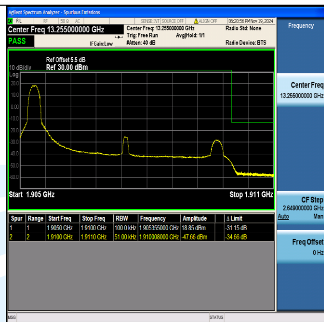
Band2 5MHz 16QAM 19175 1RB#0
