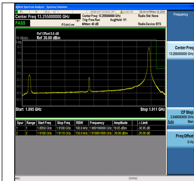
Band2 15MHz QPSK 19125 1RB#74
