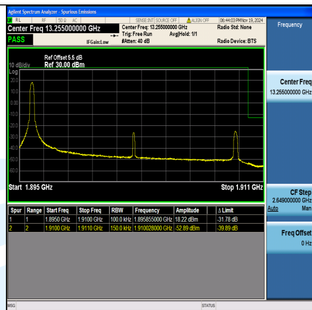
Band2 15MHz 16QAM 19125 1RB#0
