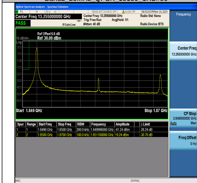
Band2 20MHz 16QAM 18700 1RB#0
