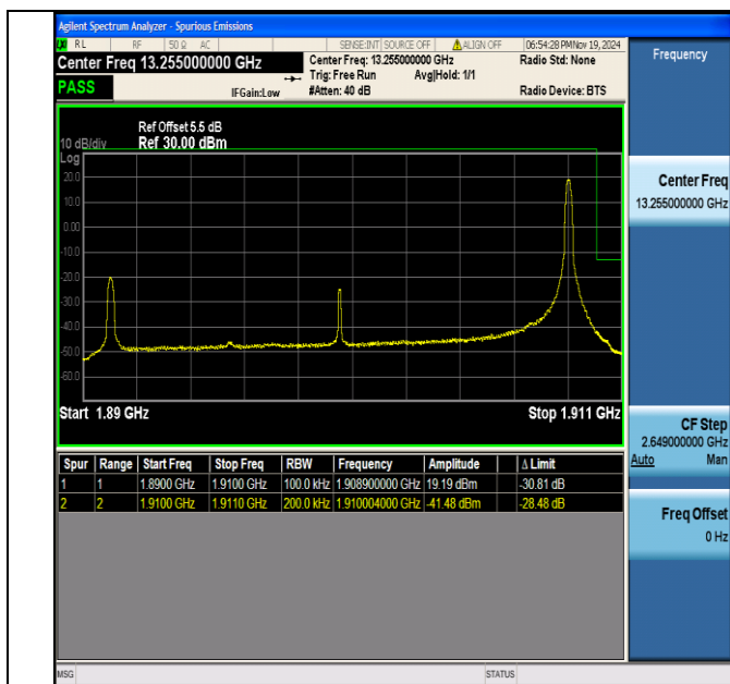
Band2 20MHz QPSK 19100 1RB#99
