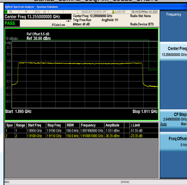
Band2 15MHz 16QAM 19125 75RB#0
