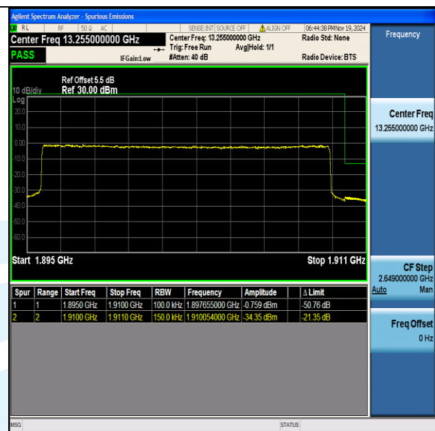
Band2 15MHz QPSK 19125 75RB#0
