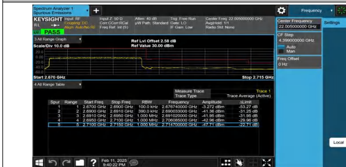
Band41-20MHz-QPSK-41490-1RB#0-PASS
