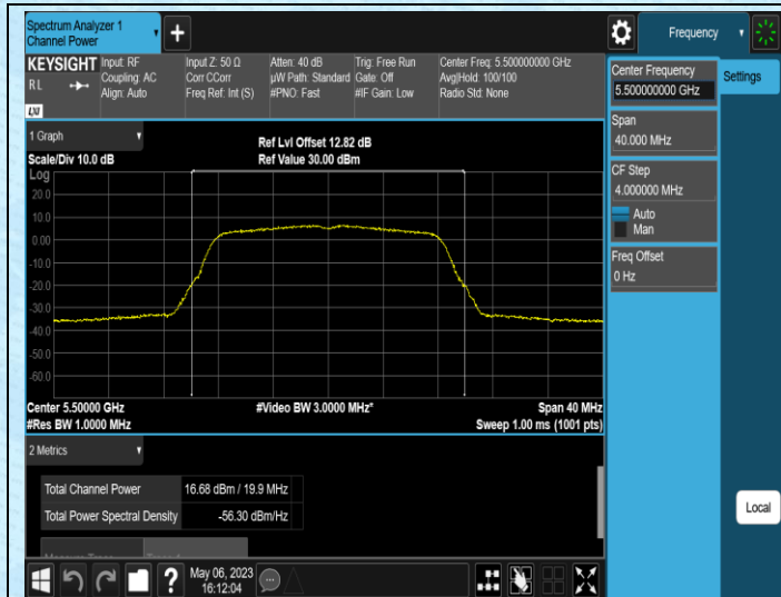
11A-Ant1-5500
