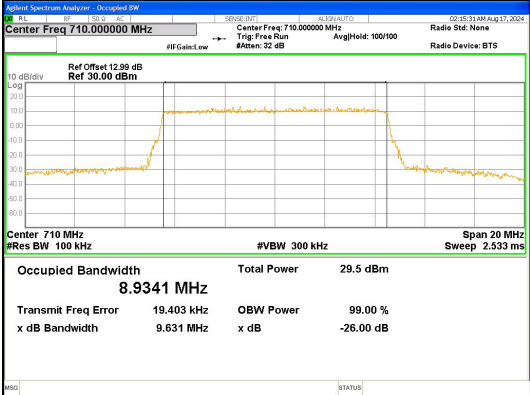
Band 17 10MHz/710.0/Mid QPSK 50@0
