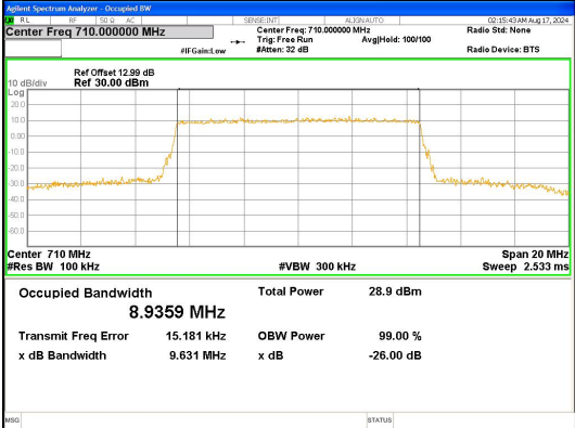
Band 17 10MHz/710.0/Mid 16QAM 50@0
