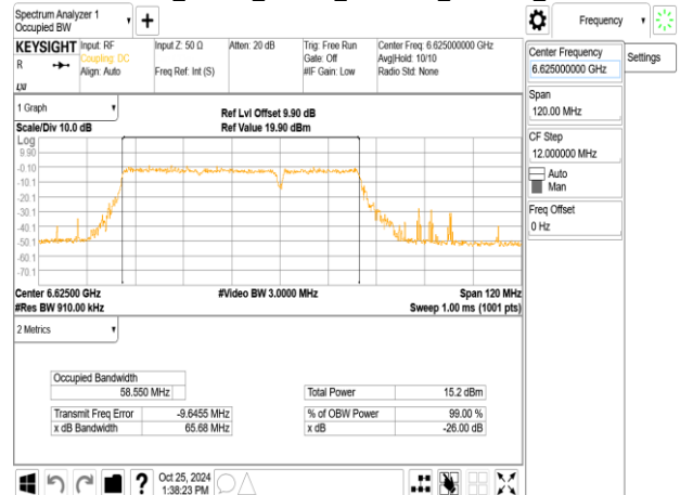
802.11be_80MHz_ChainA_6625MHz_484+242_MRU4
