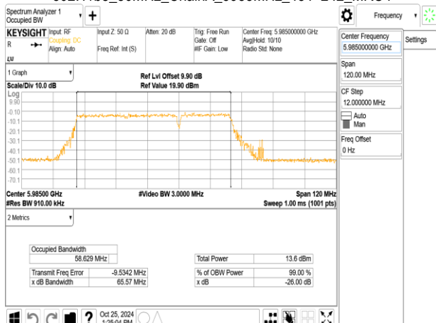
802.11be_80MHz_ChainA_5985MHz_RU484_65
