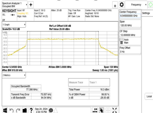
802.11be_80MHz_ChainA_6545MHz
