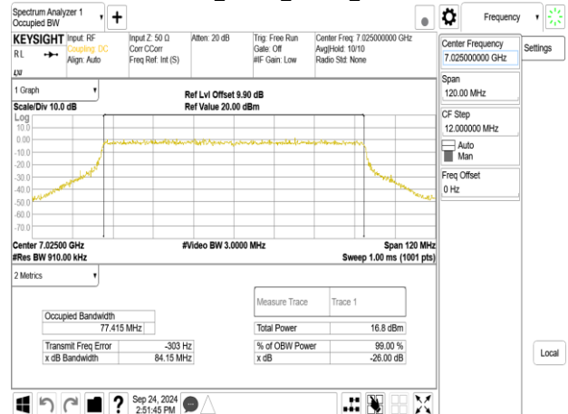
802.11be_80MHz_ChainA_7025MHz
