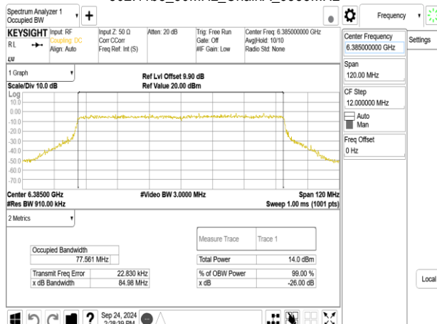
802.11be_80MHz_ChainA_6385MHz_484+242_MRU1
