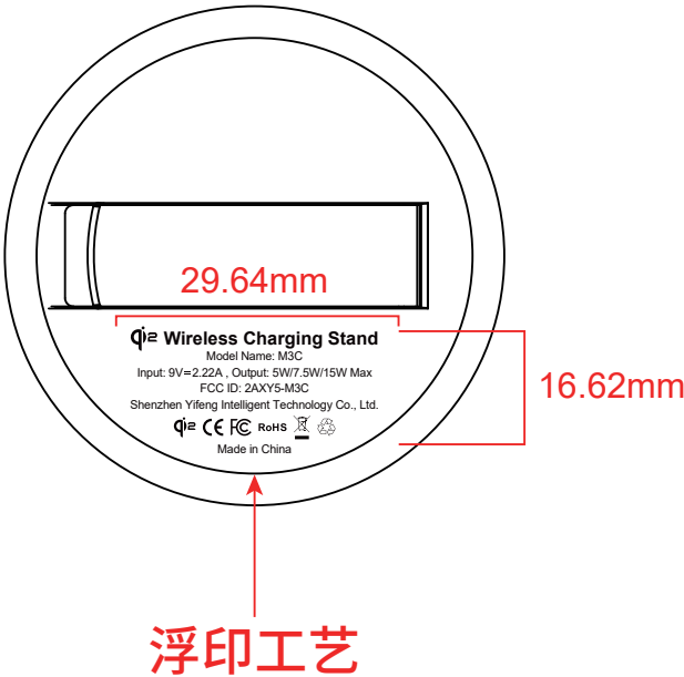
背面
