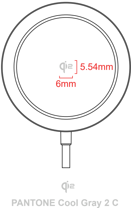
正面
