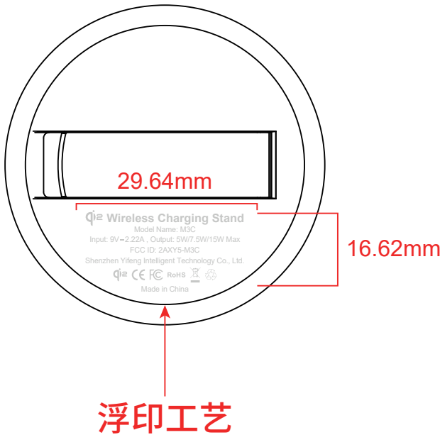
背面
