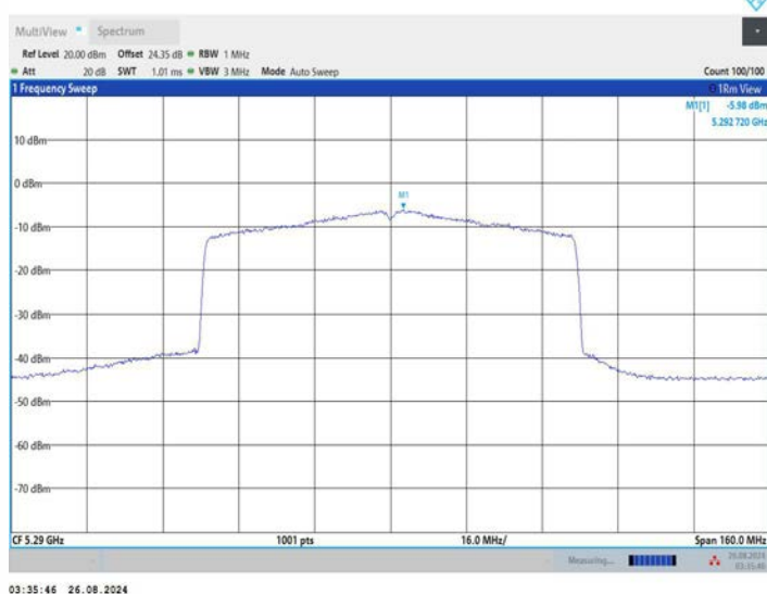
11AX80MIMO_Ant3_5290
