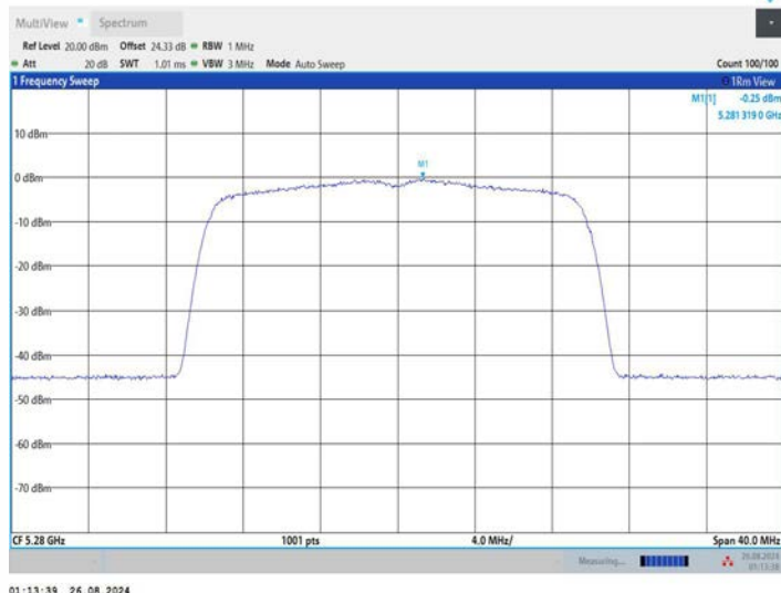
11AX20MIMO_Ant2_5280
