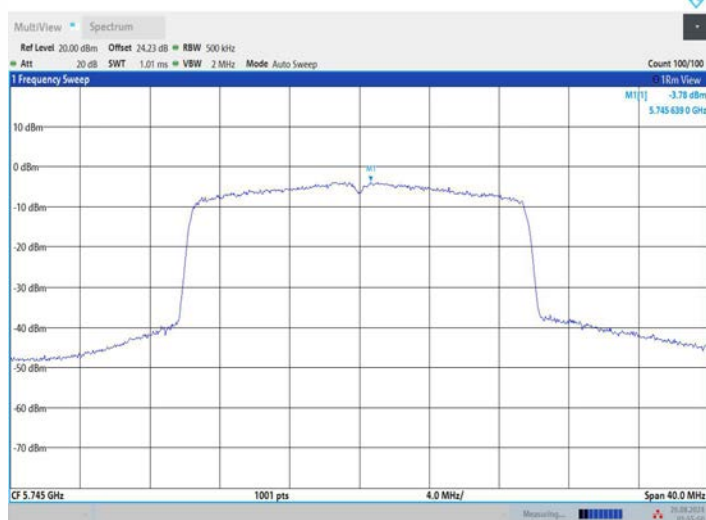
11AX20MIMO_Ant2_5745
