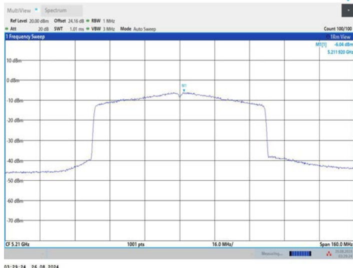
11AX80MIMO_Ant3_5210
