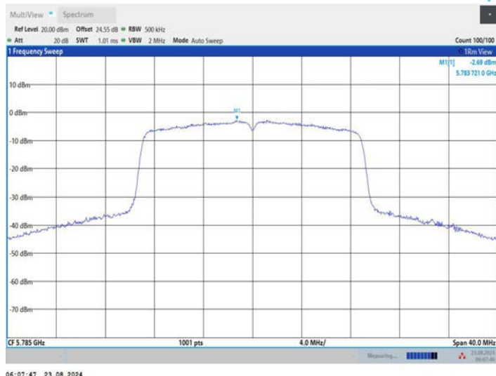
11AC20MIMO_Ant3_5785
