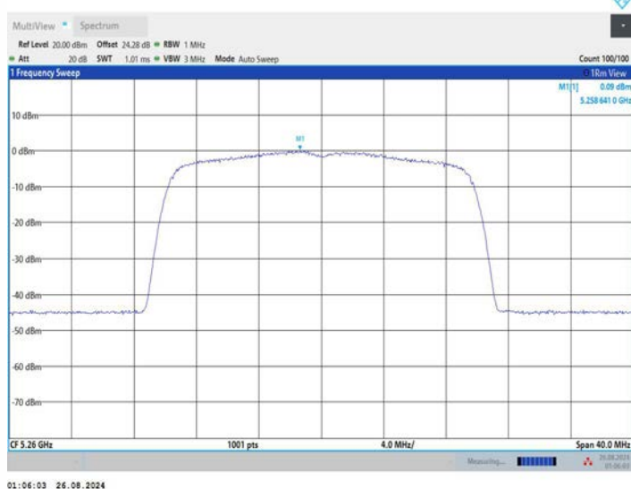
11AX20MIMO_Ant2_5260
