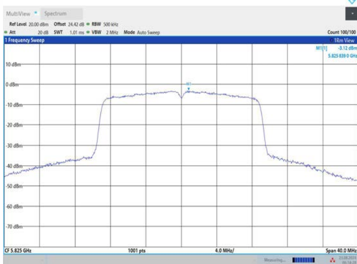
11AC20MIMO_Ant3_5825
