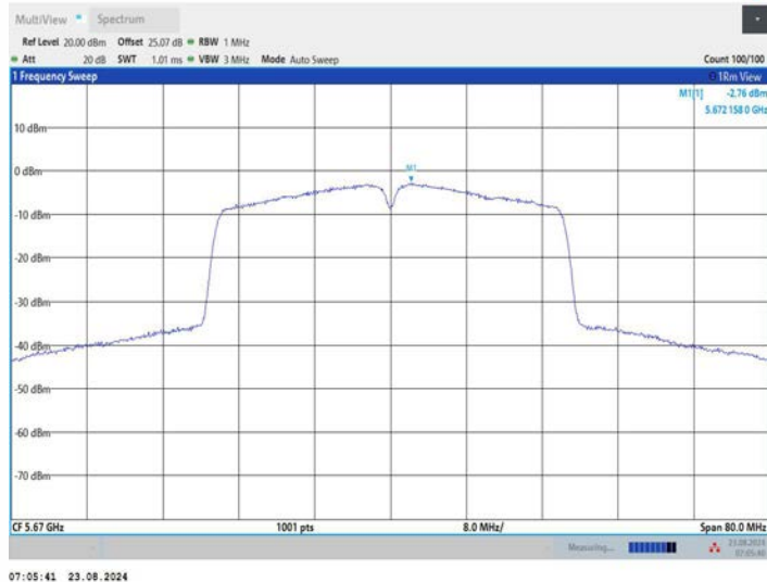
11AC40MIMO_Ant3_5670
