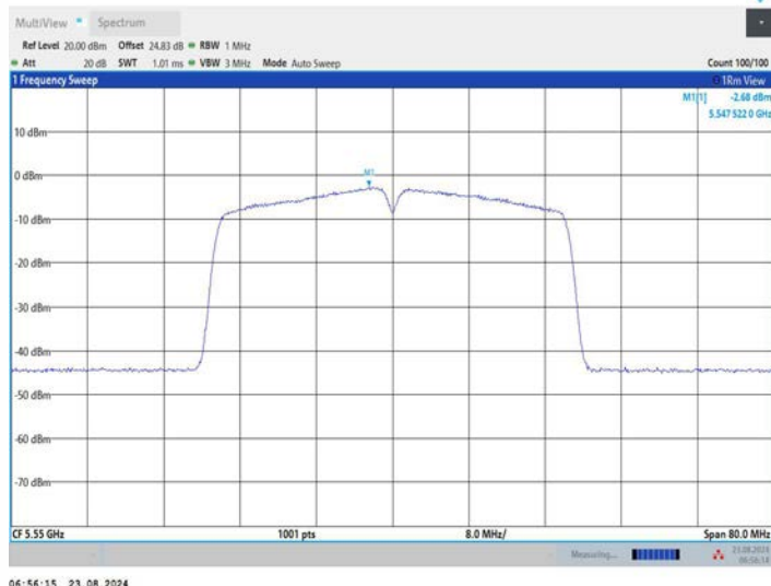
11AC40MIMO_Ant2_5550
