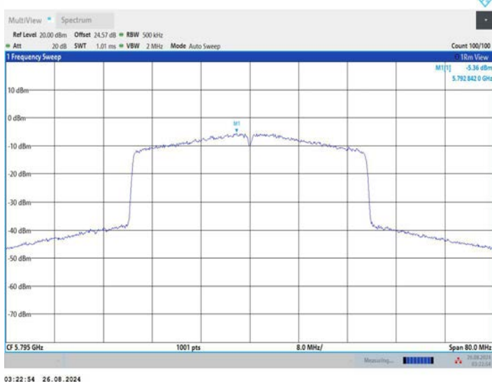
11AX40MIMO_Ant3_5795
