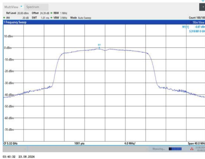
11AC20MIMO_Ant3_5320
