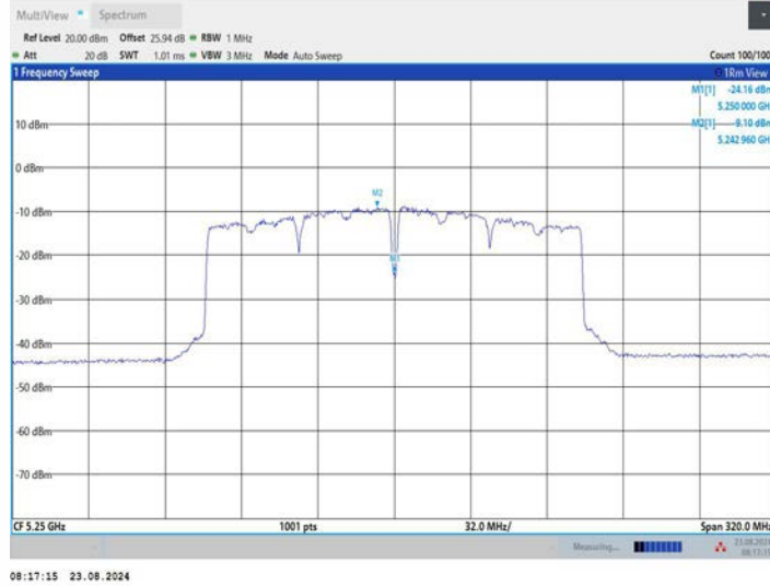
11AC160MIMO_Ant3_5250_UNII-1
