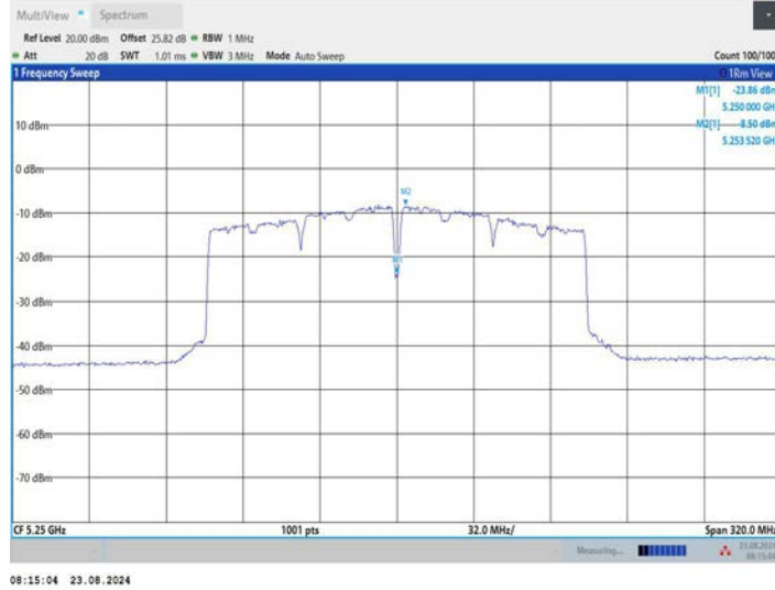
11AC160MIMO_Ant2_5250_UNII-2A
