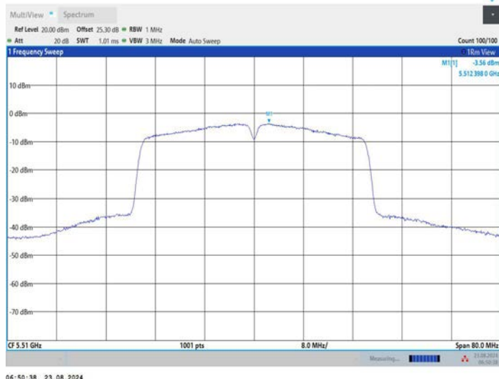
11AC40MIMO_Ant3_5510
