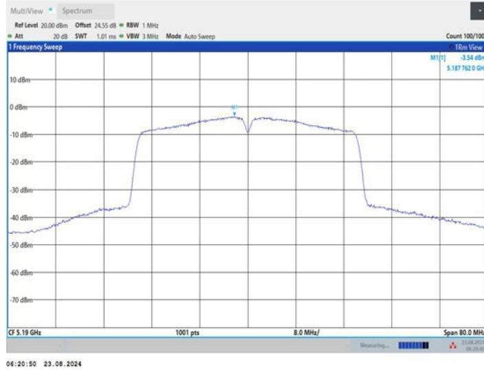
11AC40MIMO_Ant3_5190
