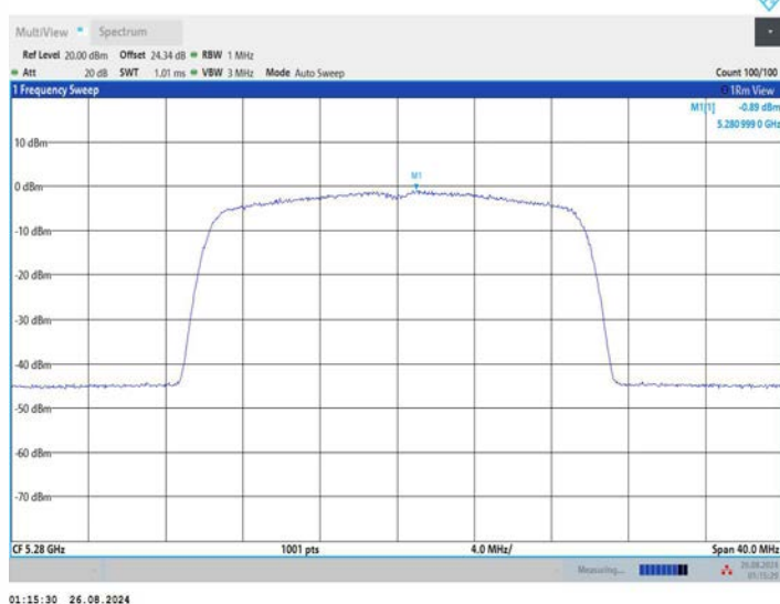
11AX20MIMO_Ant3_5280
