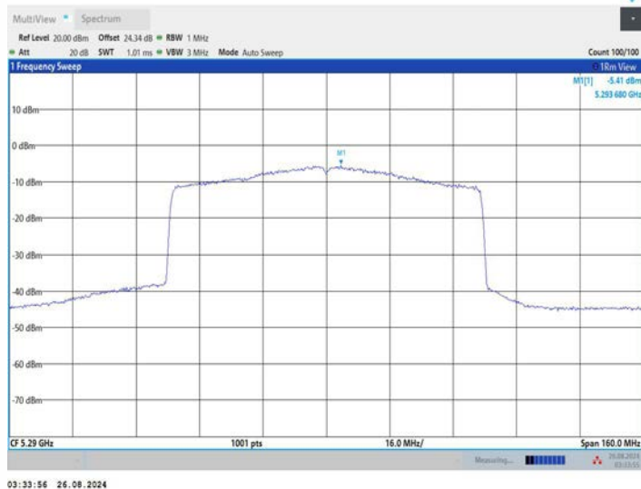
11AX80MIMO_Ant2_5290
