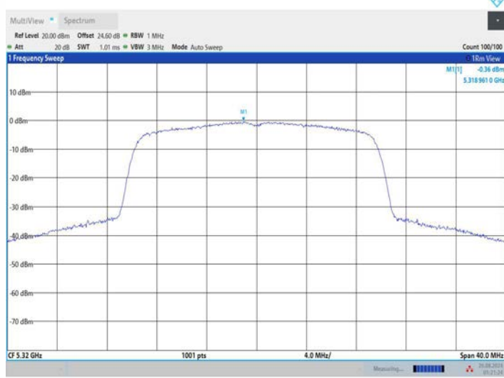
11AX20MIMO_Ant2_5320
