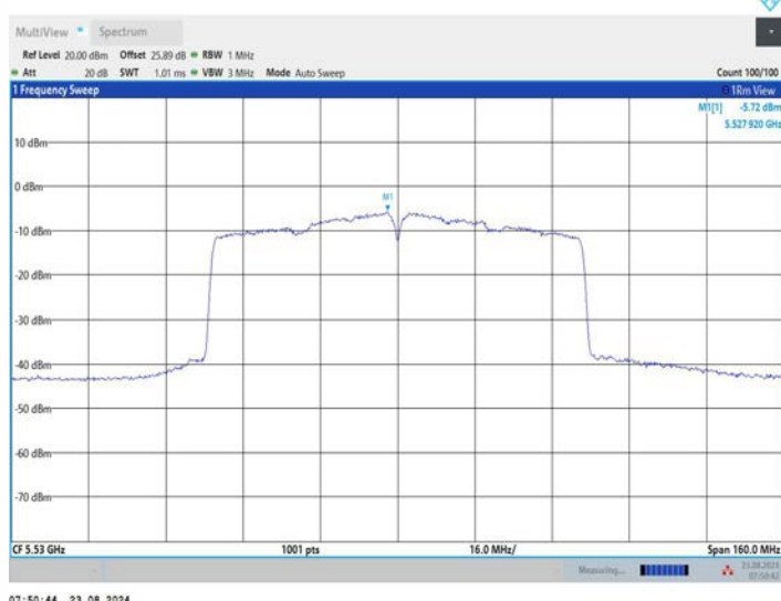
11AC80MIMO_Ant3_5530
