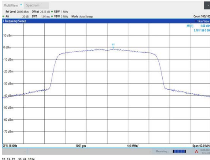
11BE20MIMO_Ant3_5180
