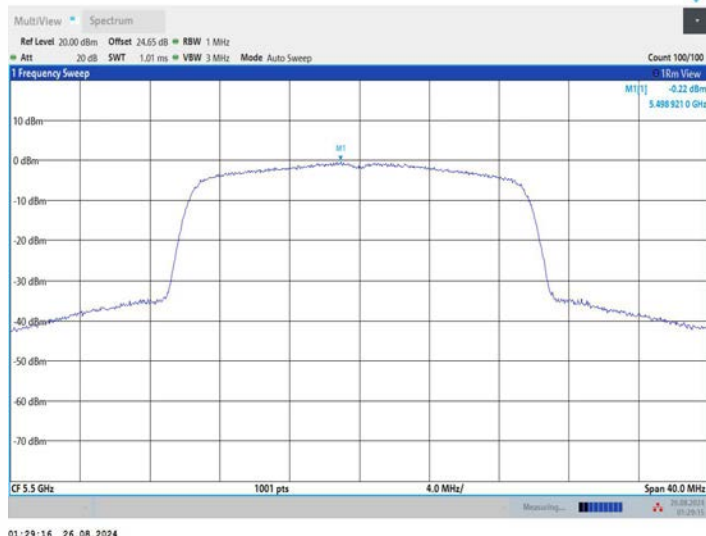
11AX20MIMO_Ant2_5500
