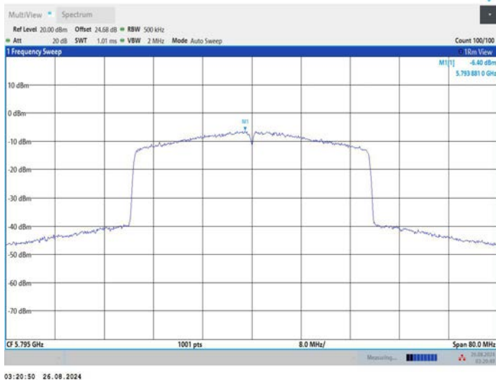
11AX40MIMO_Ant2_5795
