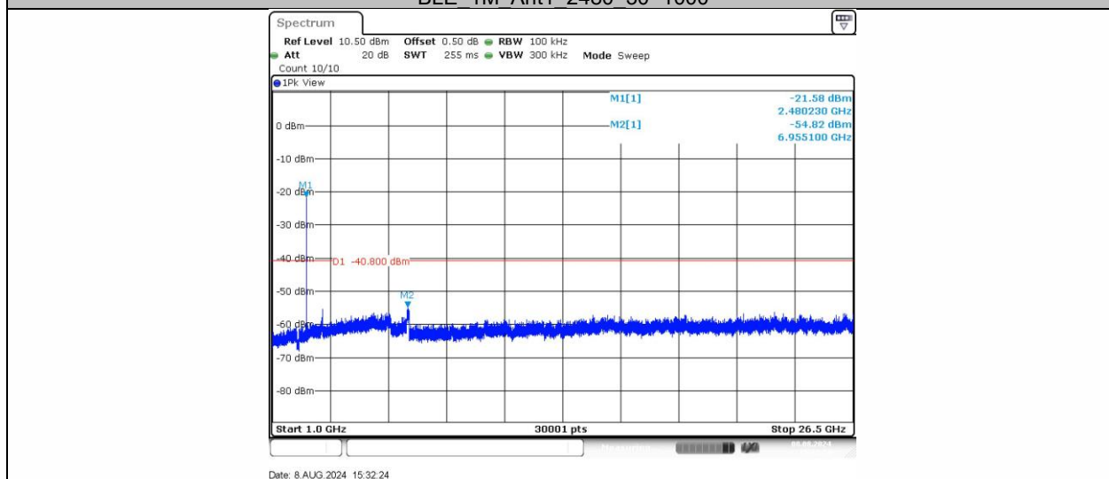
BLE_1M_Ant1_2480_1000~26500
