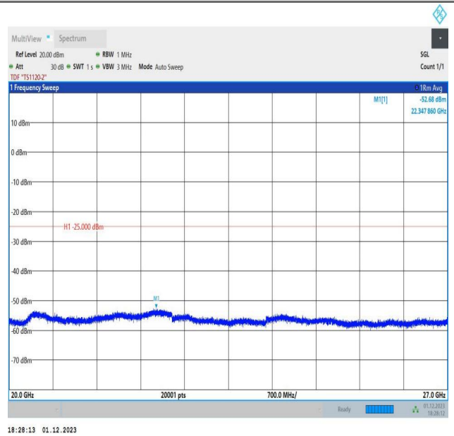
7-7-20MHz-10MHz-QPSK-QPSK-21051-21195-1RB#99-0RB# 0-20000~27000MHz-PASS
