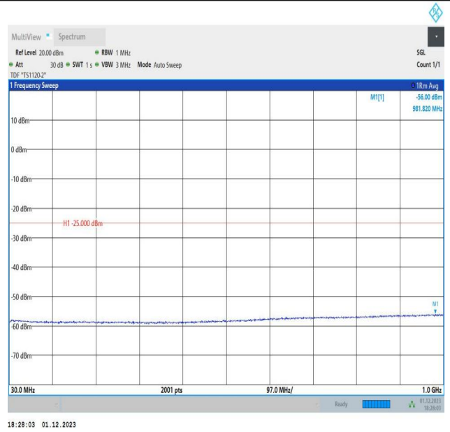
7-7-20MHz-10MHz-QPSK-QPSK-21051-21195-1RB#99-0RB# 0-30~1000MHz-PASS
