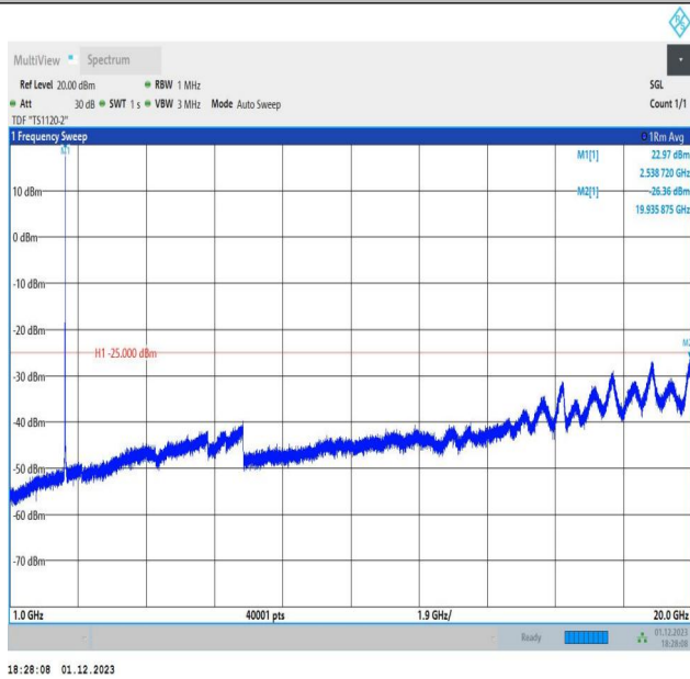
7-7-20MHz-10MHz-QPSK-QPSK-21051-21195-1RB#99-0RB# 0-1000~20000MHz-PASS
