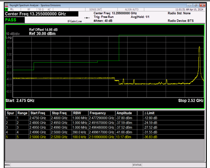
Band7_20MHz_64QAM_20850_1RB#99
