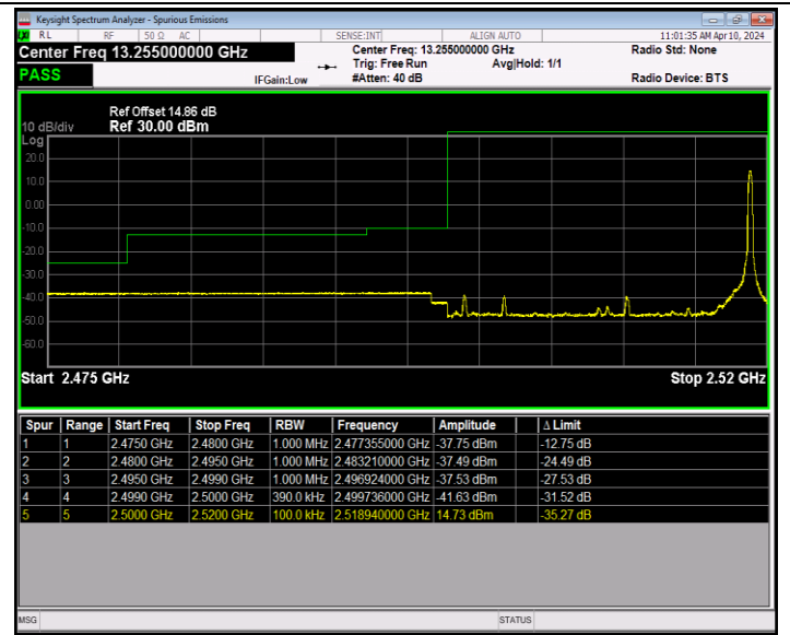
Band7_20MHz_16QAM_20850_1RB#99
