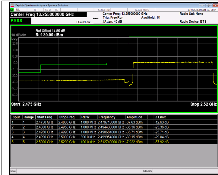
Band7_20MHz_64QAM_20850_100RB#0
