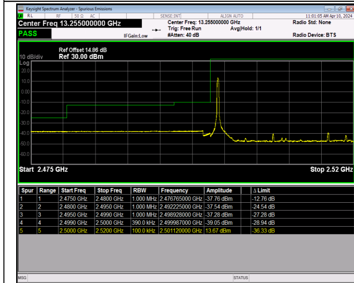
Band7_20MHz_64QAM_20850_1RB#0
