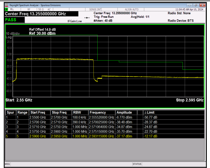
Band7_20MHz_16QAM_21350_100RB#0
