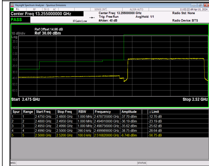
Band7_20MHz_16QAM_20850_100RB#0
