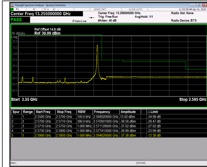
Band7_20MHz_16QAM_21350_1RB#99
