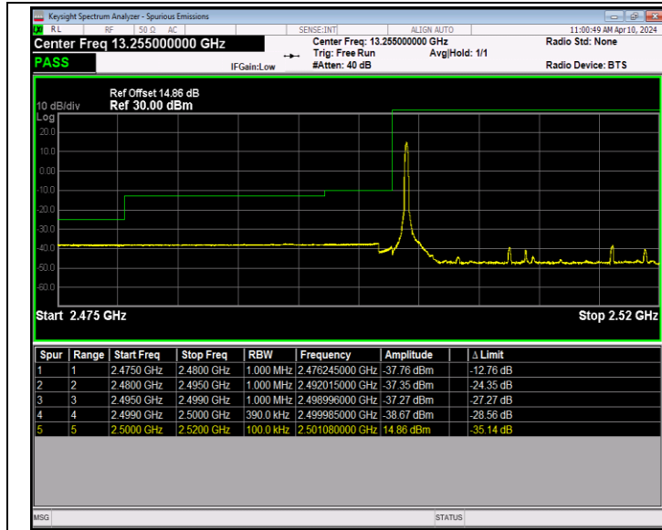
Band7_20MHz_16QAM_20850_1RB#0
