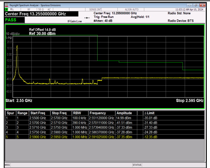
Band7_20MHz_16QAM_21350_1RB#0
