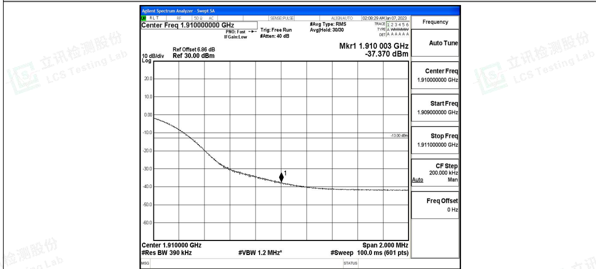
Band2-20MHz-16QAM-19100-100RB#0
