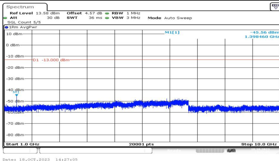
Band12-1.4MHz-QPSK-23017-1RB#0-Range4:1000~10000MHz-PASS
