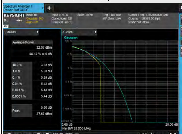
15MHz / 64QAM
