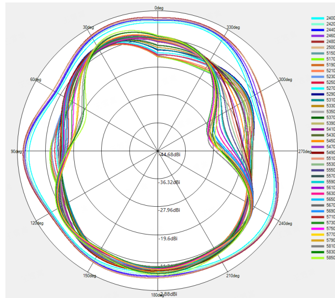
BT&WIFI-2.4G & 5G \Phi=90^\circ
