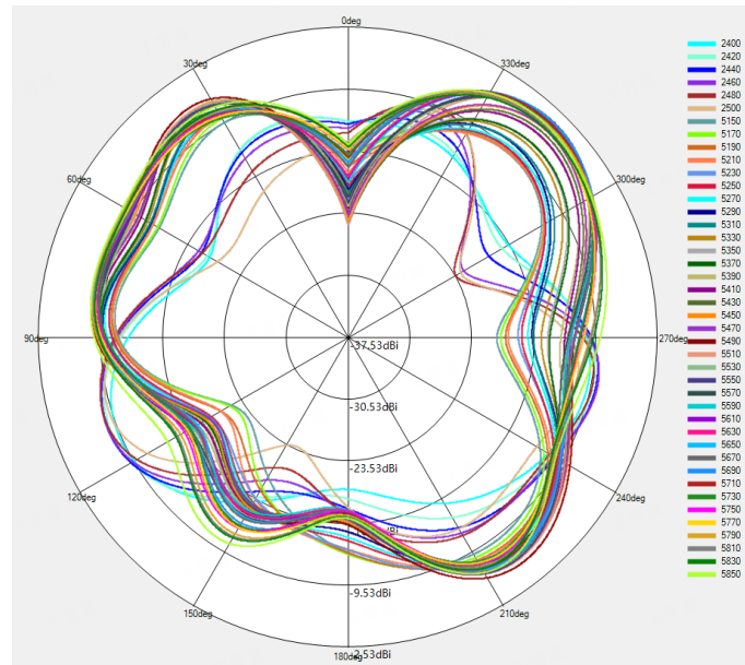
BT&WIFI-2.4G & 5G \Theta=90^\circ
