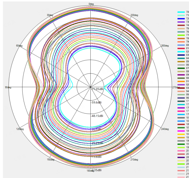
900TX/DCS1800/LTE B3 NR n3 Phi=0deg
