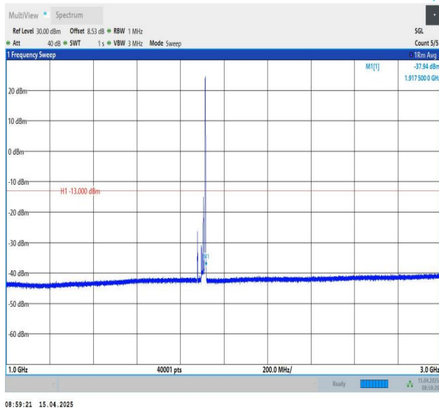
Band25-20MHz-QPSK-26590-1RB#99-1000~3000-PASS
