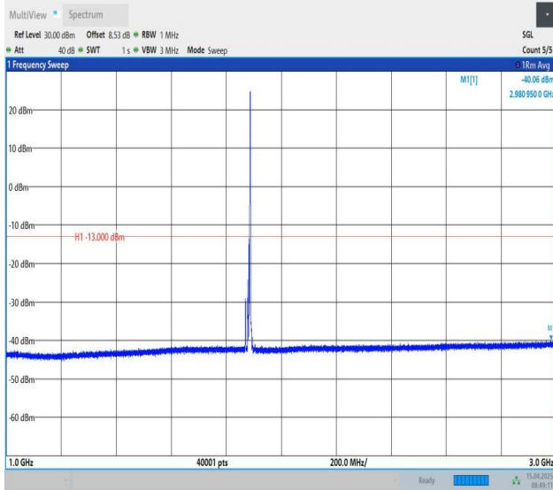
Band25-10MHz-QPSK-26365-1RB#49-1000~3000-PASS
