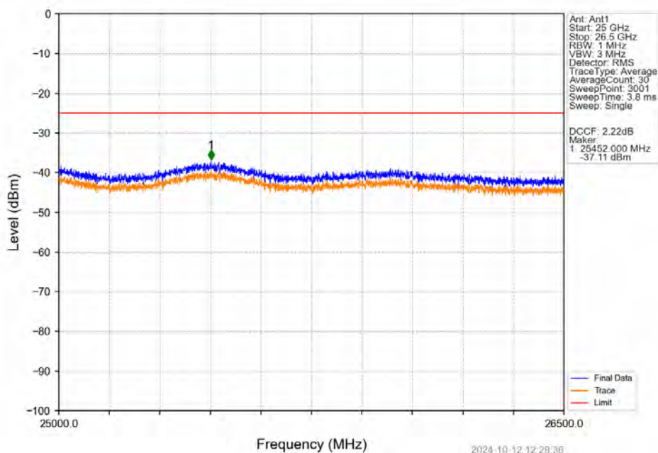
Band41_15MHz_QPSK_MCH_2593MHz_RB_1_0_NTNV
