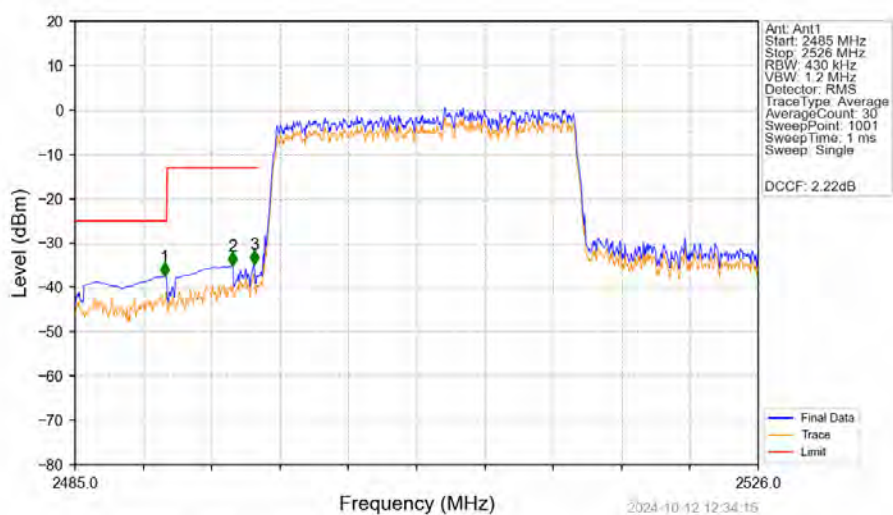
Band41_20MHz_QPSK_LCH_2506MHz_RB_100_0_NTNV
