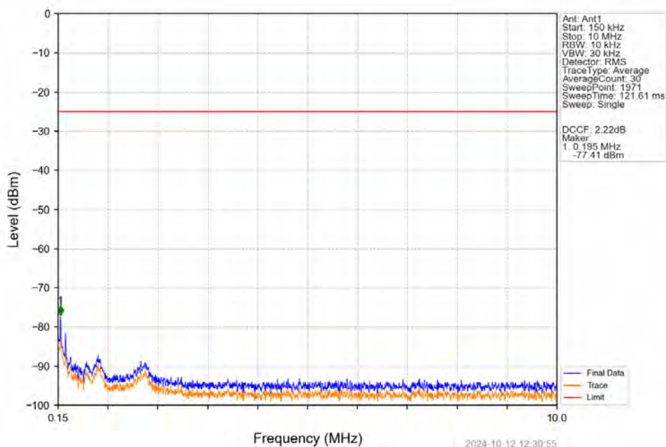
Band41_15MHz_QPSK_HCH_2682.5MHz_RB_1_0_NTNV
