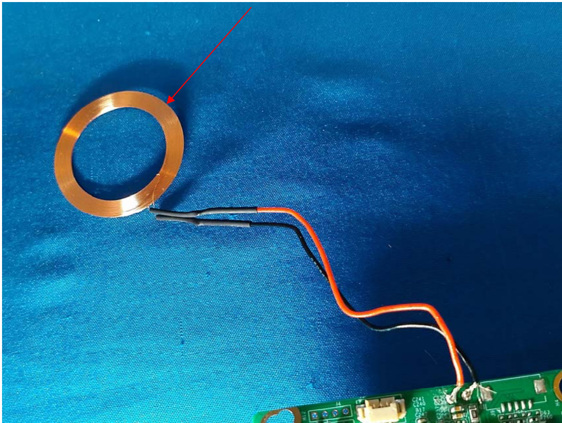
RFID(130kHz) Antenna
